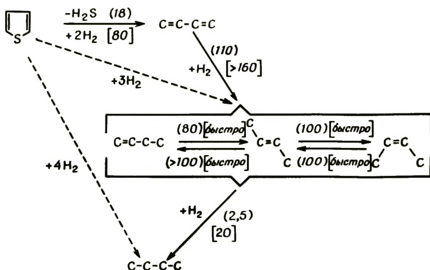
Рис. 5-2. Схема реакции гидрообессеривания тирфена [1]. Числа в скобках – приближительные скорости [ммоль/(г · с)]; в круглых скобках – для катализатора Cr 2 O 3 при температуре 415°C, в квадратных скобках – для катализатора Co – Mo/Al 2 O 3 при температуре 400°C. [Copyright by the American Chemical Society.]
