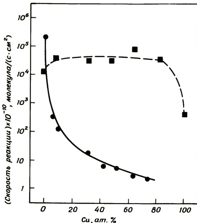
Рис. 3-27. Активность сплавных катализаторов Cu – Ni в гидрогенолизе этана до метана и дегидрогенизации циклогексана. Активность относится к скоростям реакции при 316°C. Активность в гидрогенолизе этана определяли при парциальных давлениях этана и водорода, равных 0,03 и 0,20 атм соответственно [47]. ■ дегидрогенизация циклогексана, ● гидрогенолиз этана. [ Copyright by Academic Press.]
