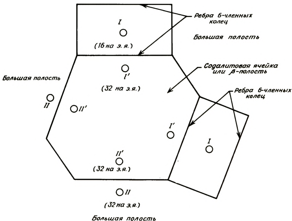
Рис. 1-35. Двумерная модель содалитовой ячейки и двух прилегающих гексагональных призм. (з.я. — элементарная ячейка.)
