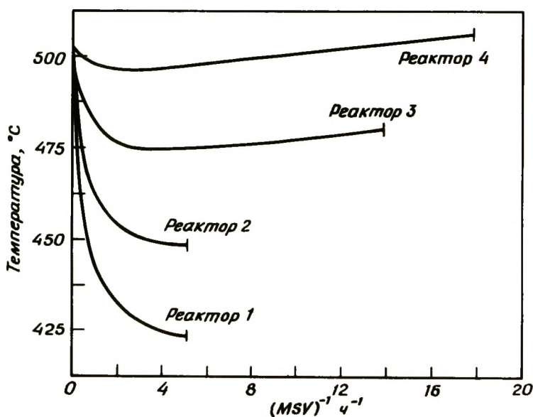
Рис. 3-74. Рассчитанные температурные профили в четырех реакторах [224].
