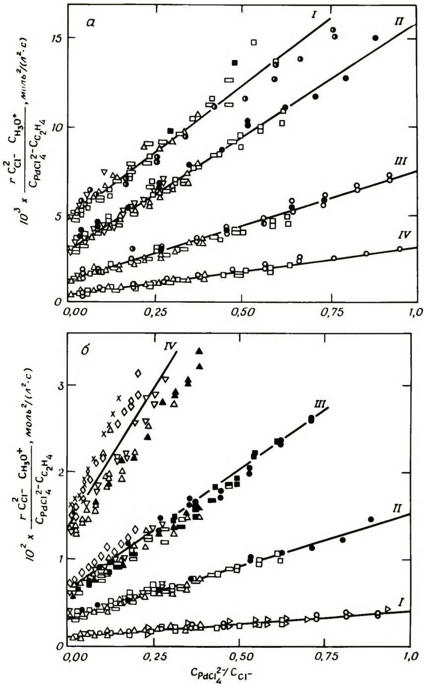
Рис. 2-10. Кинетика окисления этилена водными растворами PdCl_4^{2-} при различной ионной силе (а) и различных температурах (б). Концентрация ионов Cl^- (моль/л): \circ 0,2; \square 0,3; \square 0,4; \Delta 0,5; \nabla 0,7; \diamond 1,0; \times 1,4. Все светлые кружочки относятся к C_{H_3O^+} = 0,2 М; все темные кружочки относятся к C_{H_3O^+} = 0,5 М; \bullet C_{H_3O^+} = 0,1 М, C_{Cl^-} = 0,2 М; \bullet C_{H_3O^+} = 0,8 М, C_{Cl^-} = 0,2 М; \bullet C_{H_3O^+} = 1,0 М, C_{Cl^-} = 0,2 М; \bullet C_{H_3O^+} = 1,5 М, C_{Cl^-} = 0,2 М [13]. [Copyright by the American Chemical Society.]
