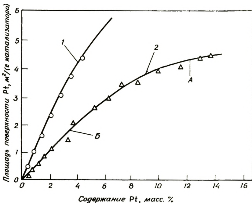
Рис. 3-35. Влияние содержания Pt и методики приготовления на размер кристаллита металла. Содержание металла изменяли путем изменения концентрации в растворе. Катализатор высушивали при 120°C, затем восстанавливали [92]. 1 — катализатор получен ионным обменом, 15 А; 2 — импрегнированный катализатор; А — область, в которой число кристаллитов постоянно, размер частиц увеличивается; Б — область, в которой размер частицы не меняется, 30 А, число частиц увеличивается. [Copyright by Academic Press.]
