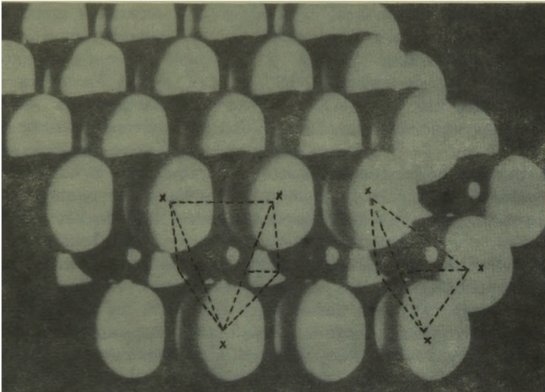
Рис. 5-11. Модель небольшого кристаллита WS_2 [326]; белые шары — ионы серы, черные — вольфрам. Стерическое препятствие адсорбции вызвано атомами серы, обозначенными на рисунке крестиками. [Copyright by Academic Press.]
