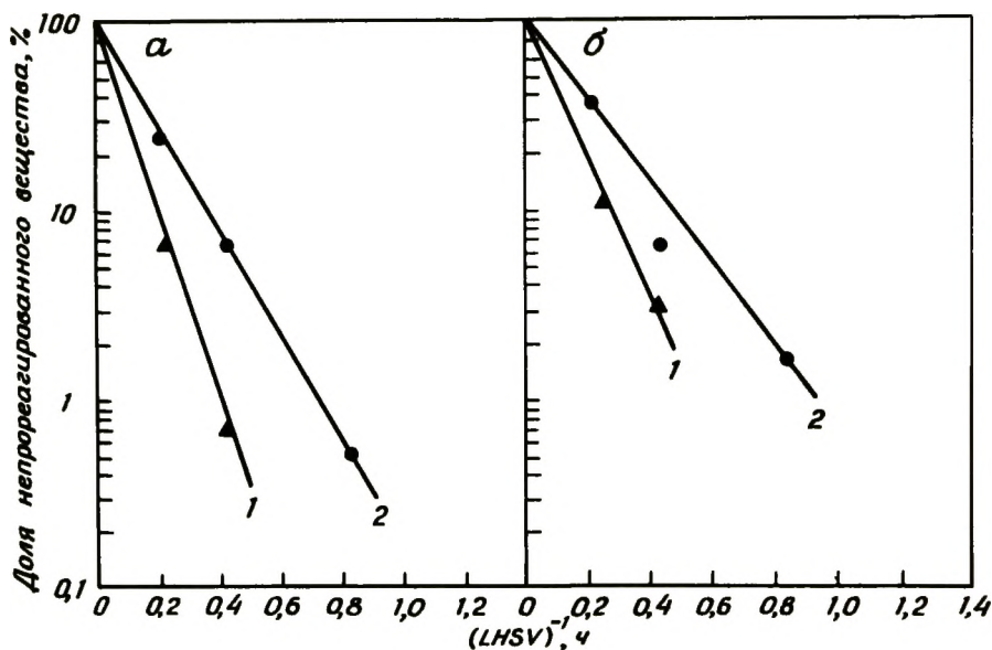
Рис. 5-25. Реакция деметаллизации первого порядка нефтяных остатков (Агха Джари) в присутствии включений марганца при 398°C и 137 атм [63]. а) — ванадий: 1) k = 11,5 \text{ ч}^{-1} ; 2) k = 6,43 \text{ ч}^{-1} ; б) — никель: 1) k = 8,54 \text{ ч}^{-1} ; 2) k = 5,06 \text{ ч}^{-1} . ● частицы 14 — 30 меш; ▲ частицы 60 — 80 меш. [Copyright by the American Chemical Society.]
