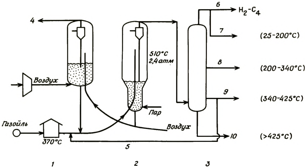
Рис. 1-1. Схема потоков в процессе каталитического крекинга. 1 – регенератор; 2 – реактор; 3 – разделитель; 4 – отходящий газ к испарителю (675°C, 2,1 атм); 5 – рецикл; 6 – легкий газ H_2 - C_4 ; 7 – катализат, фракция 25 – 200°C; 8 – легкий катализат, фракция 200 – 340°C; 9 – тяжелый катализат, фракция 340 – 425°C; 10 – остаточная фракция > 425°C.
