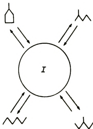
Рис. 3-51. Схема реакции изомеризации C 6 -парафина на поверхности металла. I — пятичленное кольцо на поверхности.
