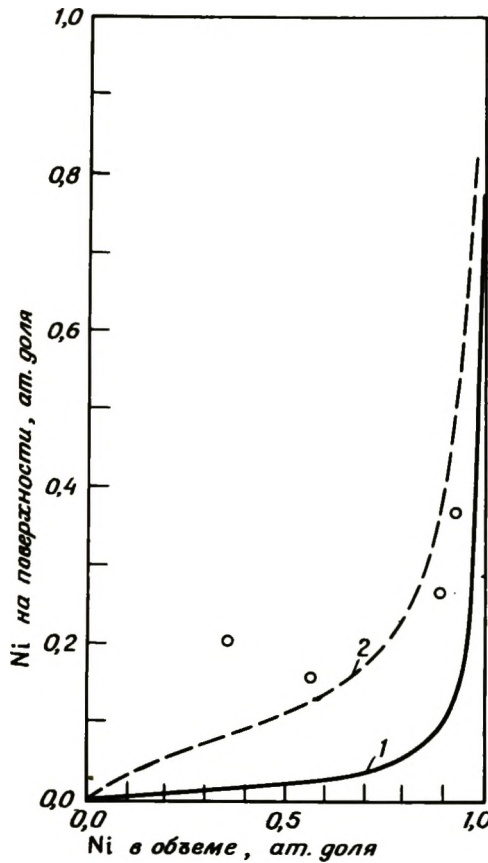
Рис. 3-21. Предположительный состав поверхности пленок из Cu – Ni; расчеты были сделаны для поверхности [111] гранецентрированной кубической решетки с использованием параметров взаимодействия металлов \Delta H_{\text{sub}} = 10 \text{ кТ} и \Omega = 0,1 \text{ кТ} . 1 – для свободной поверхности; 2 – для поверхности с адсорбированным на ней водородом, с \Delta H_{\text{ads}} = 5 \text{ кТ} и \Omega = 0,1 \text{ кТ} [40]. \circ данные из [41].
