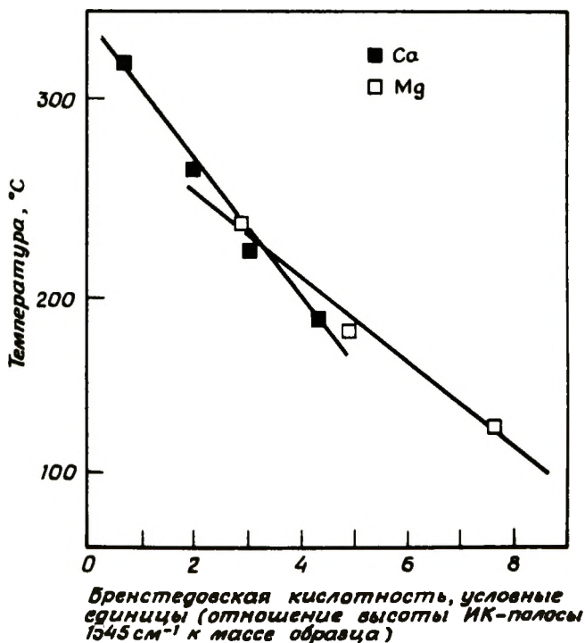
Рис. 1-45. Корреляция между каталитической активностью (измеренной как температура, необходимая для 20% изомеризации о-ксилола) и брэнстедовской кислотностью кальциевого и магниевго фожазитов. Более низкая температура обозначает более высокую активность [95]. [Copyright by Academic Press.]
