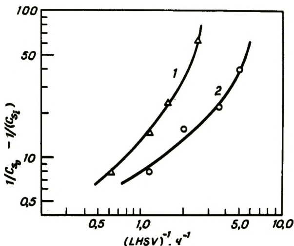
Рис. 5-23. Данные по конверсии, полученные Парскосом и сотр. [59] и представленные в виде графика для проверки контактной эффективности в реакции второго порядка. 1 — 416°C; 2 — 393°C. [Copyright by the Chemical Society.]
