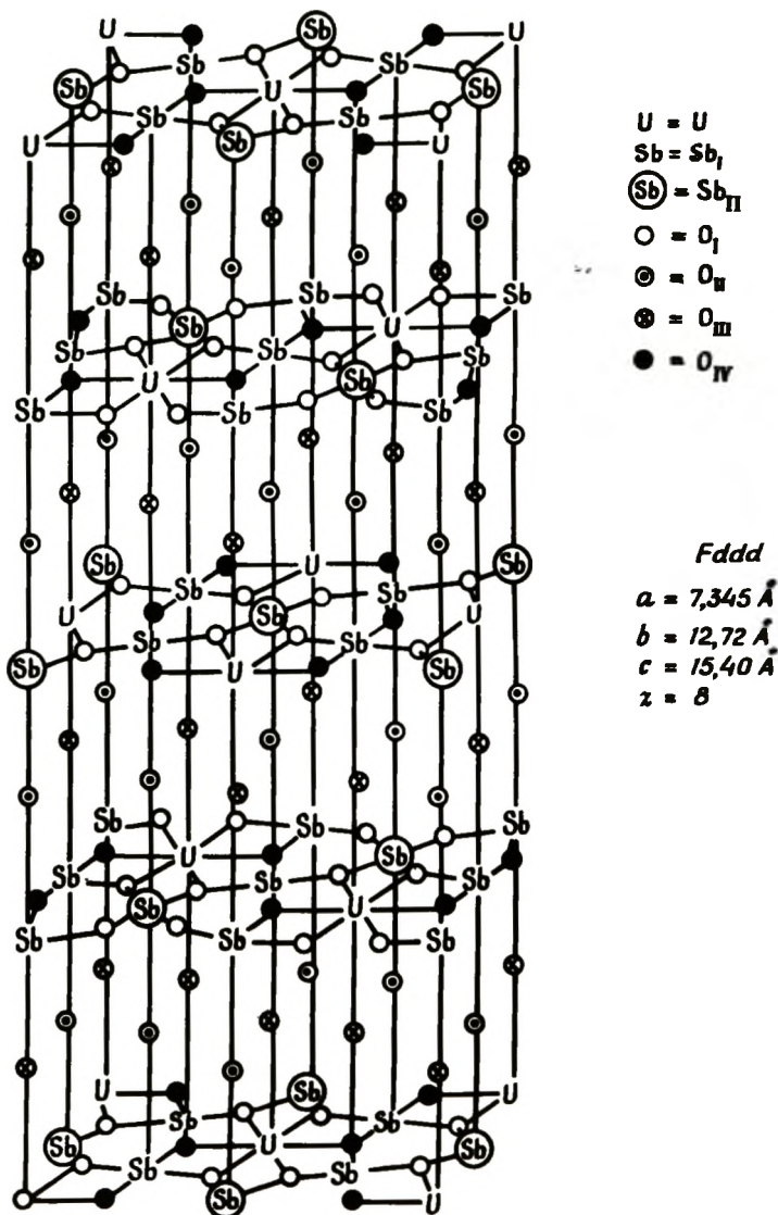
Рис. 4-21. Элементарная ячейка фазы \text{USb}_3\text{O}_{10} в катализаторе U – Sb окислительно-го аммонолиза [13]. [Copyright by Academic Press.]
