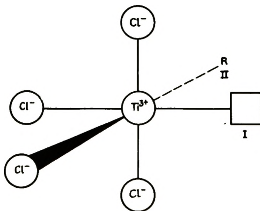
Рис. 2-36. Центр на грани слоя \alpha - TiCl_3 по Косси и Арльману. R — алкильная группа (растущая полимерная цепь); □ — незаполненное координационное место.
