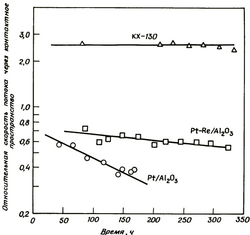
Рис. 3-66. Данные по активности и стабильности катализаторов Pt/Al 2 O 3 , Pt — Re/Al 2 O 3 и (полиметаллический компонент)/Al 2 O 3 (KX-130) в реформинге парафиновой нефти с образованием продукта с постоянным содержанием октана [217]. Данные получены на пилотной установке с использованием ближневосточного сырья (парафинистая нефтя), общее давление 9,2 атм, средняя температура 499°C, октановое число чистого продукта 102,5 (дорожное октановое число).
