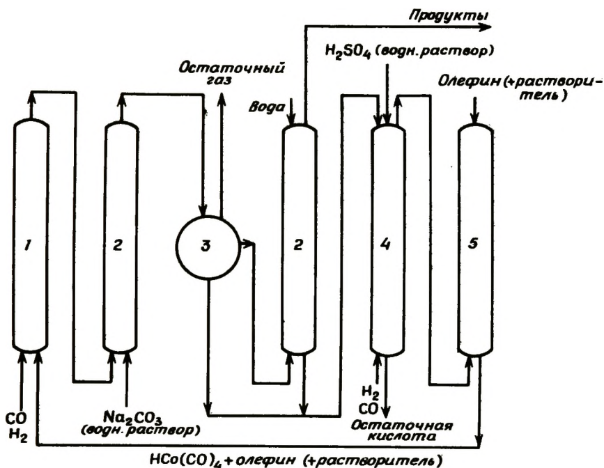
Рис. 2-20. Схема процесса оксосинтеза по Кульману [34]. 1 – реактор гидроформирования; 2 – экстракционная колонна; 3 – фазовый сепаратор; 4 – регенератор-скруббер; 5 – поглотительная колонна.
