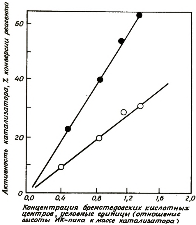
Рис. 1-41. Зависимость каталитической активности алюмосиликатов при изомеризации o -ксилола от содержания Al_2O_3 [68]. Образцы нагревались до 500^\circ C (●) и до 425^\circ C (○). [Copyright by Academic Press.]
