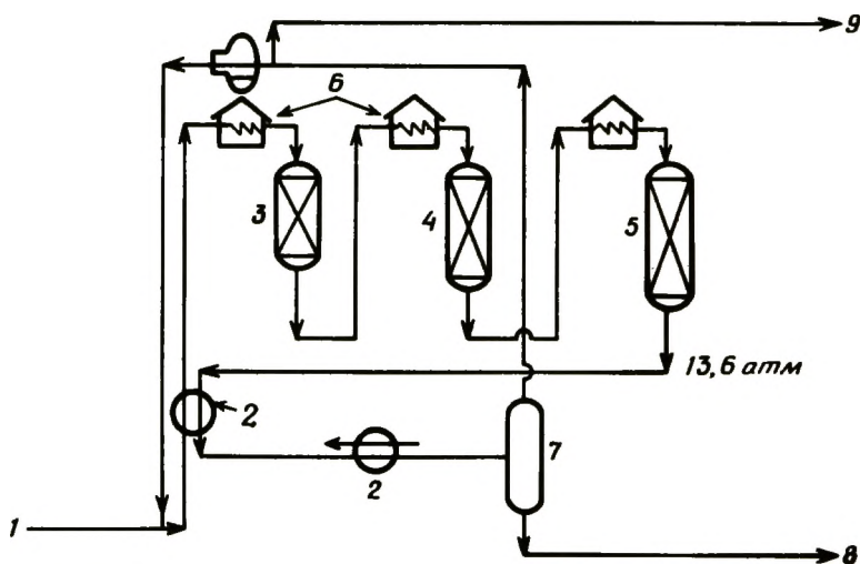
Рис. 3-3. Схема установки для реформинга с тремя реакторами. 1 — нефтя (25000 баррелей в день); 2 — теплообменники; 3, 4, 5 — реакторы; 6 — подогрев сырья; 7 — разделение продуктов (10,2 атм); 8 — на отгонку легких фракций; 9 — низшие газы.
