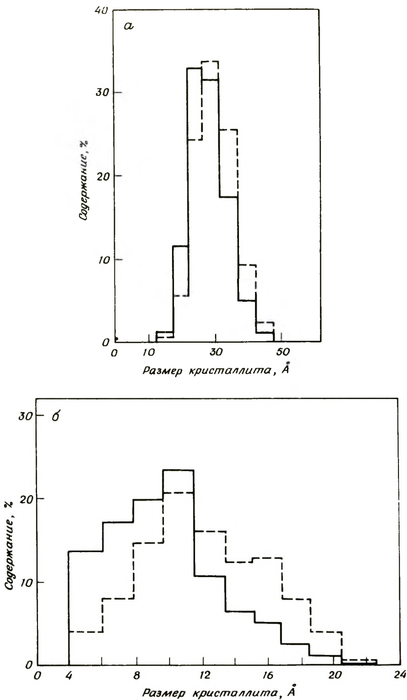
Рис. 3-37. Распределение кристаллитов Pt по размеру, определенное с помощью электронной микроскопии. а – 2,5 масс.% Pt на силикагеле [97]; б – 2,83 масс.% Pt на \gamma -Al 2 O 3 [98]. Оба катализатора приготавливали путем пропитки платинахлористоводородной кислотой и восстановления водородом; сплошная линия относится к распределению по числу, штриховая линия – к распределению по площади поверхности. [ а – Copyright Academic Press; б – Copyright by Johnson Matthey and Company Limited.]
