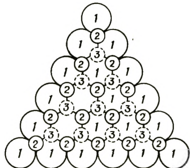
Рис. 3-40. Монослой плотноупакованных сфер (1): 2 и 3 — места дополнительных слоев.
