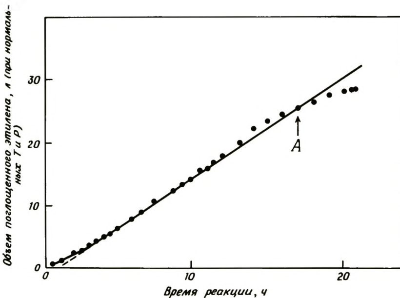
Рис. 2-26. Полимеризация этилена в реакторе периодического действия [41]. Условия: T = 40^\circ\text{C} , 200 мл циклогексена, 0,525 ммоль/л \gamma\text{-TiCl}_3 , 5,25 ммоль/л \text{Al}(\text{C}_2\text{H}_5)_2\text{Cl} , P_{\text{этилен}} = 643 мм рт. ст. Точке А соответствует 17% взвеси; выход составляет 2020 г полиэтилена на 1 г \text{TiCl}_3 .
