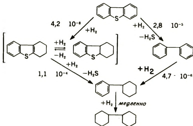
Рис. 5-3б. Схема реакции гидрообессеривания дибензотиофена [8а]. Катализатор — сульфидированный \text{Co} - \text{Mo} / \text{Al}_2\text{O}_3 при температуре 300°C и давлении 102 атм; числа над стрелками — константы скорости реакции псевдопервого порядка (в \text{м}^3 / \text{кг катализатора} \cdot \text{с} ) [8а].
