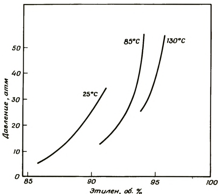
Рис. 2-15. Пределы взрываемости этилен-кислородных смесей [19].
