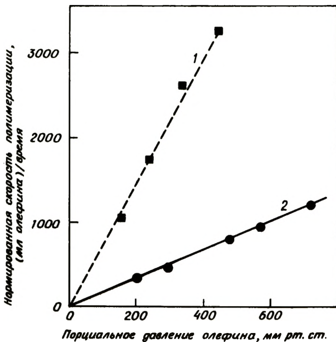
Рис. 2-29. Зависимость скорости полимеризации от парциального давления олефина [40]. 1 – этилен, 50°C, [TiCl_2] = 1,27 ммоль/л, [AlEt_3] = 9,8 ммоль/л, 110 мл синароля; 2 – пропилен, 56°C, [TiCl_3] = 14 ммоль/л, [AlEt_3] = 81 ммоль/л, 100 мл синароля. [Copyright by Academic Press.]
