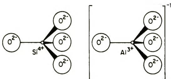
Рис. 1-29. Первичные блоки структуры цеолита.
