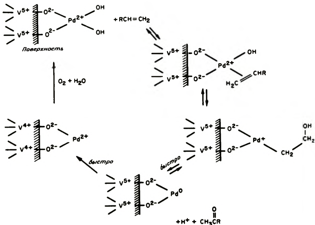
Рис. 4-8. Механизм вакер-процесса, катализируемого V 2 O 5 , промотированного палладием [6]. [Copyright by Academic Press.]
