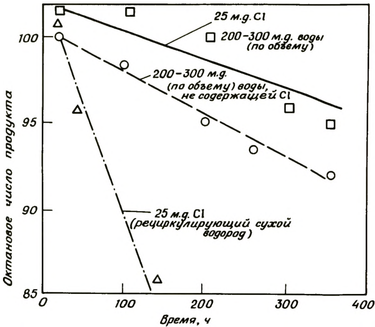
Рис. 3-67в. Влияние содержания хлора в сырье и воды в потоке рециркулирующего водорода на активность и стабильность реформинга [222]. Условия исследования в пилотной установке: температура 496°C, LHSV = 3 ч -1 H 2 /НС = 6, давление 150 атм.
