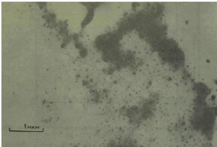
Рис. 2-27. Электронно-микроскопический снимок полипропилена через 6 мин после начала реакции. Частицы TiCl_3 с размерами от 100 до 1000 Å распределены в массе полимера [45].
