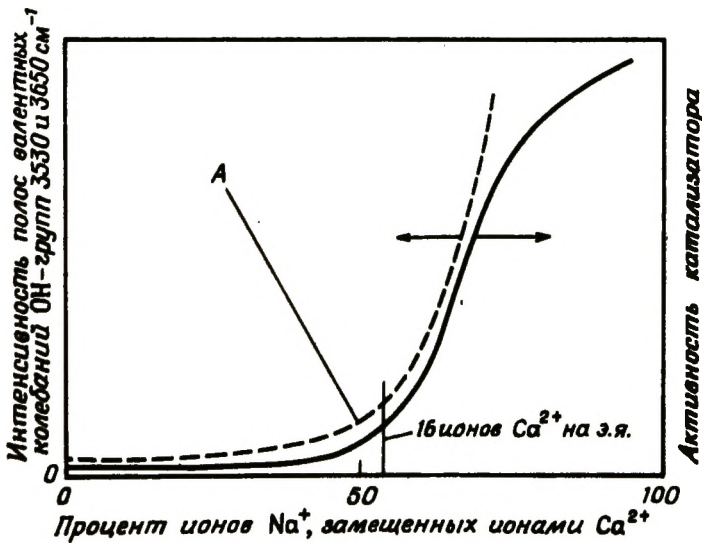
Рис. 1-42. Качественная корреляция между активностью в крекинге кумола и концентрацией доступных брэнстедовских центров в катализаторе — цеолите Y. А — точка, при которой впервые наблюдается взаимодействие пиридина с катионами Ca^{2+} .
