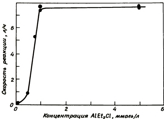
Рис. 2-24. Влияние концентрации алкилалюминия на скорость полимеризации этилена [41]. T = 40^{\circ}\text{C} ; P = 760 мм рт. ст.; [\text{TiCl}_3] = 5 ммоль/л.
