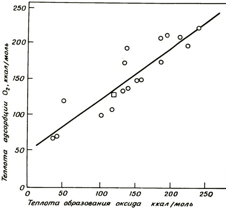
Рис. 3-11. Корреляция между начальной теплотой адсорбции кислорода на напыленных металлических пленках и теплотой образования наиболее устойчивых оксидов при 25°C [11]. Квадратные точки для азот-танталовой системы.
