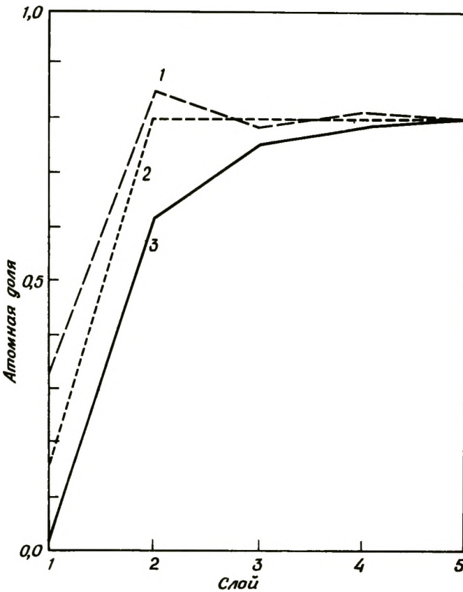
Рис. 3-22. Профили изменяющегося теоретического состава в процессе сегрегации на поверхности (111) г.-ц.к. решетки бинарного сплава. Разность теплот испарения составляет \Delta H_{\text{sub}} = 10 kT ; атомная доля в объеме — 0,8 [40]. 1) \Omega/kT = 0,1 ; 2) идеальный состав; 3) \Omega/kT = 0,1 .
