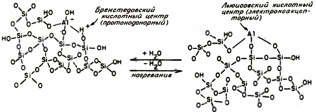
Рис. 1-28. Конверсия брэнстедовского кислотного центра в льюисовский при дегидратации алюмосиликата.
