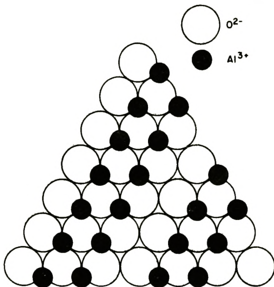
Рис. 3-49. Структура и положения катиона в \theta\text{-Al}_2\text{O}_3 .
