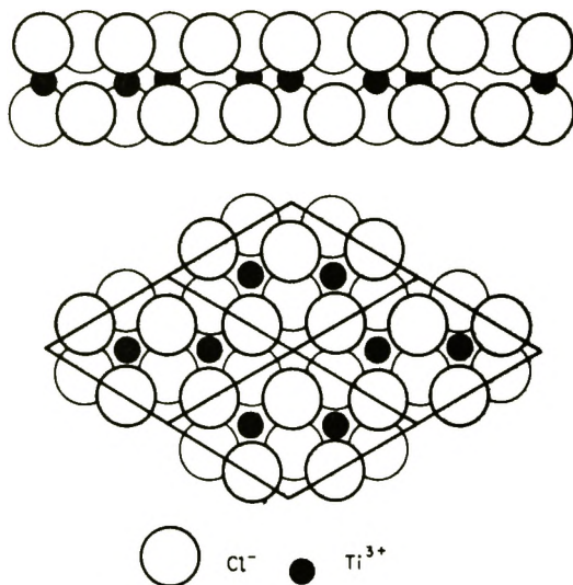
Рис. 2-32. Расположение ионов в слоистой структуре \alpha\text{-TiCl}_3 .
