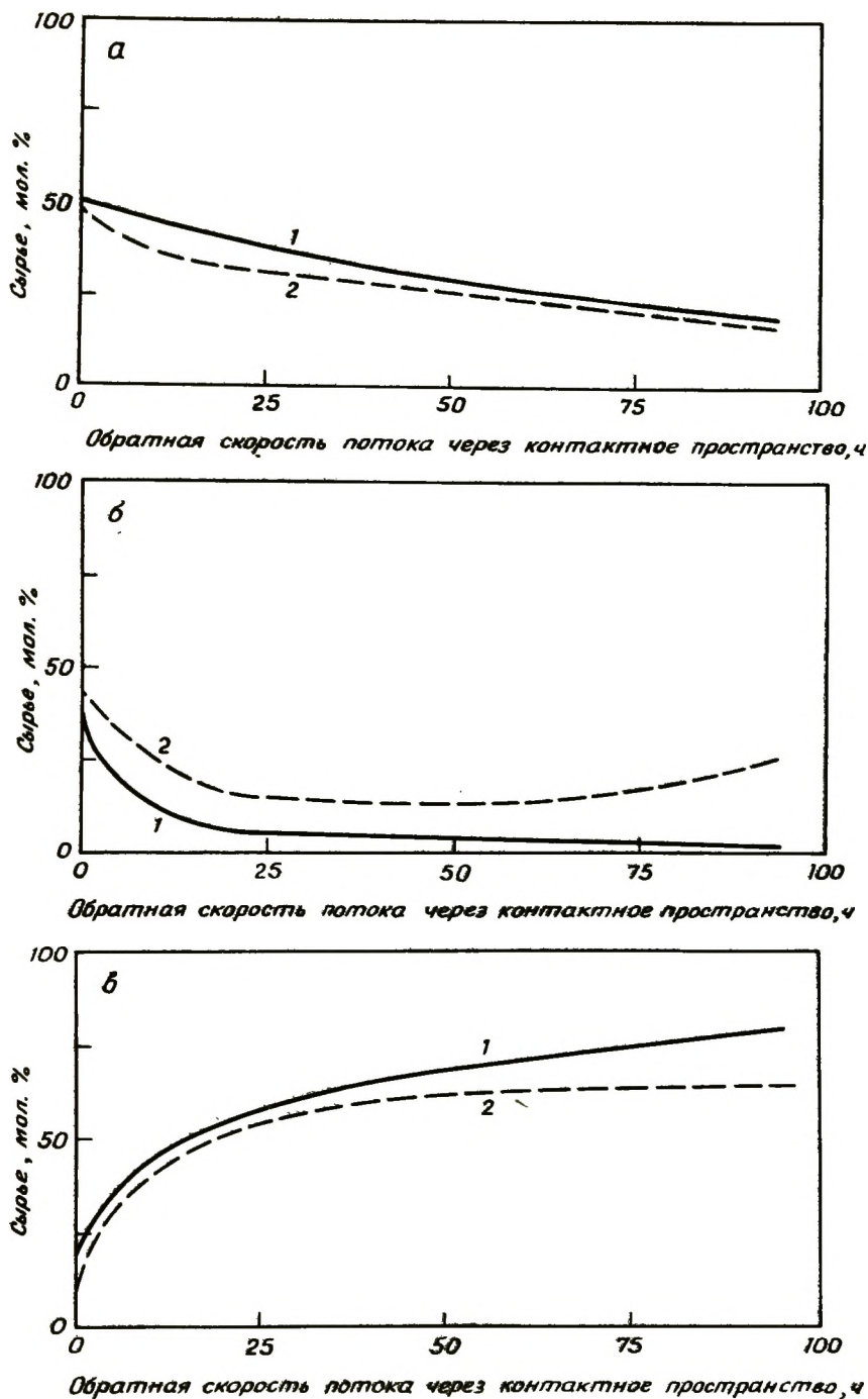
Рис. 3-72. Сравнение конверсии (1), рассчитанной с помощью общей параметрической модели, использующей среднее значение k для каждой группы реакций, с конверсией (2), предсказанной Крейном и сотр. [6]. а — парафины; б — нафтенны; в — ароматические углеводороды.
