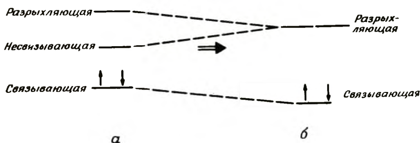
Рис. 1-9. Энергетические уровни, соответствующие открытой трехцентрковой связи (а) и замкнутой трехцентрковой связи (б).
