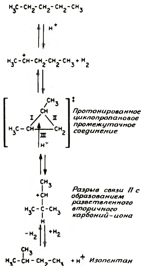
Рис. 1-5. Механизм изомеризации n -пентана в изопентан.
