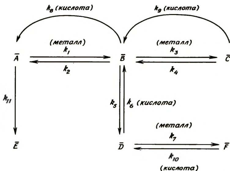
Рис. 3-68. Превращения метилциклопентана, катализируемые смесью больших монофункциональных частиц катализатора [226, 227]. A – метилциклопентан, B – метилциклопентен, C – метилциклопентадиен, D – циклогексен-1, E – продукты гидрогениза, F – бензол.
