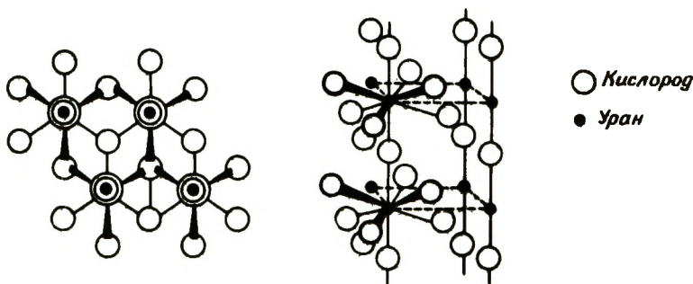
Рис. 4-18. Структура UO_3 [61].
