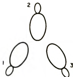
Рис. 1-8. Двухэлектронная трехорбитальная система B_2H_6 .
