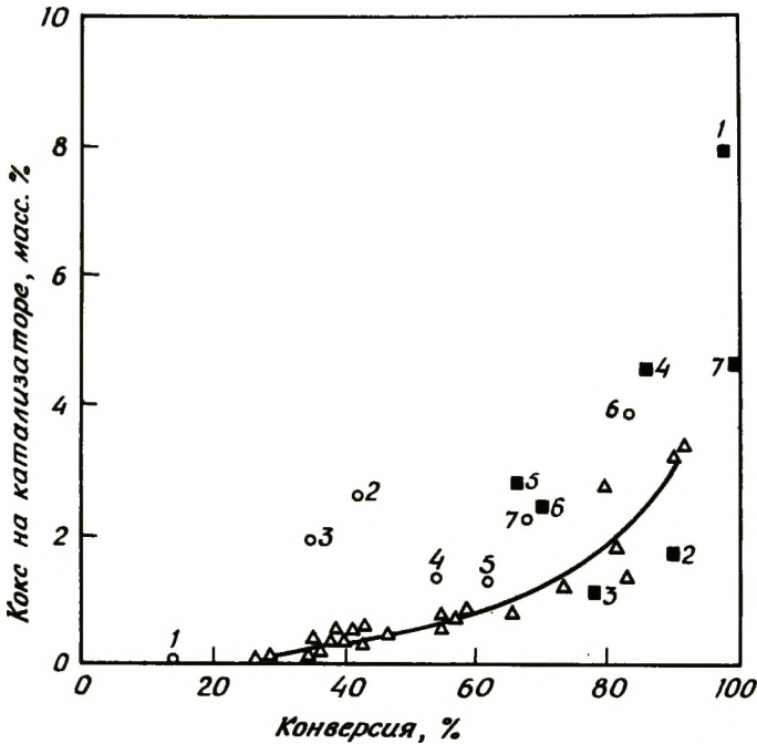
Рис. 1-22. Количество коксообразования при крекинге чистых углеводородов.
