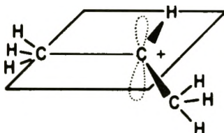
Рис. 1-3. Структура "классического" вторичного пропилкарбоний-иона.
