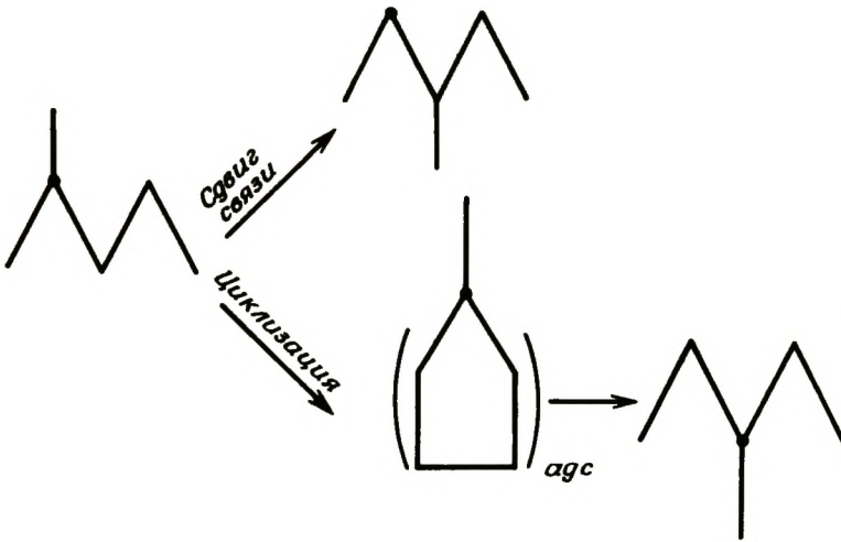
Рис. 3-54. Сдвиг связи и циклическая изомеризация 2-метилпентана-2- 13 С.
