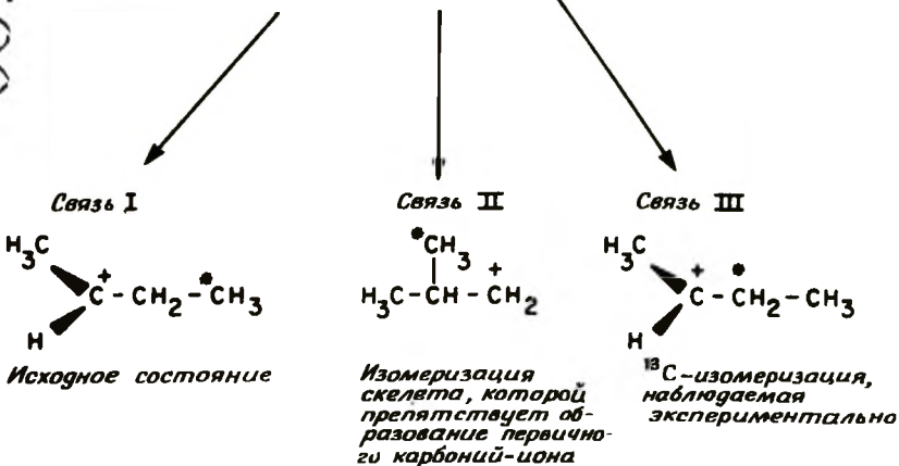
Рис. 1-4. Структура протонированного циклопропанового кольца, образованного из классического втор-бутилкарбоний-иона и карбоний-ионов, образовавшихся в результате разрыва указанных связей С - С.
