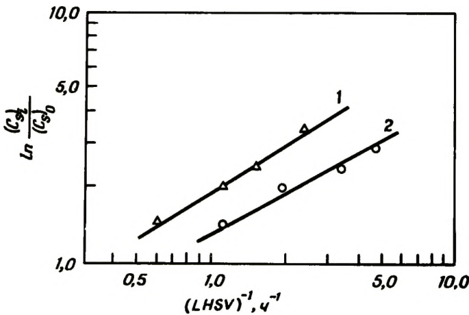
Рис. 5-22. Данные по конверсии, полученные Параскосом и сотр. [59] и представленные в виде графика для проверки контактной эффективности в реакции первого порядка. 1 – наклон 0,62, температура 416°С; 2 – наклон 0,53, температура 393°С. [Copyright by the American Chemical Society.]
