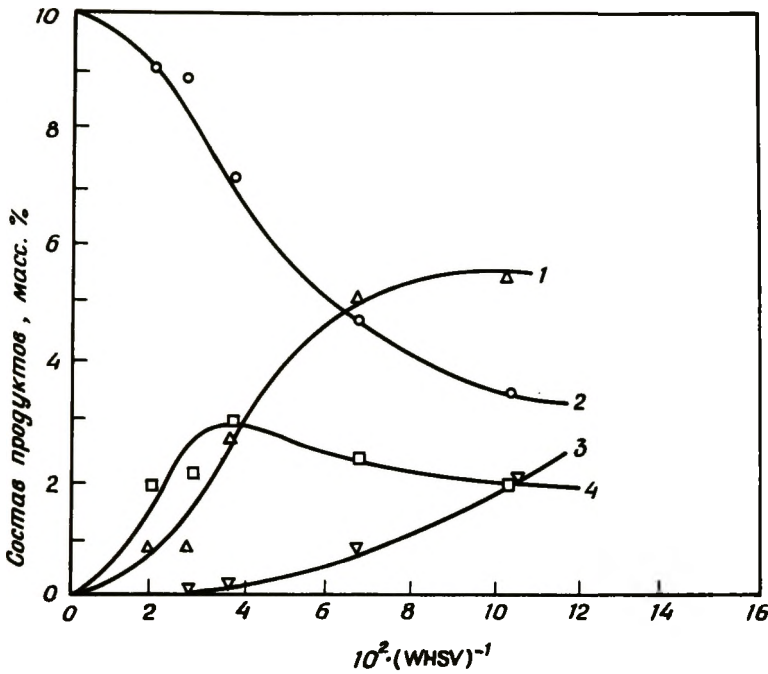
Рис. 3-53. Состав продуктов реакции 2-метилпентана на Pt, нанесенной на некислотный оксид алюминия. Условия реакции: температура 440°C, давление 9,5 атм; мольное соотношение \text{H}_2 : 2-метилпентан = 4; катализатор — 0,5 масс.% Pt на некислотном оксиде алюминия [136]. 1) 0,20 × (3-метилпентан); 3) бензол; 4) метилциклопентан. (WHSV см. рис. 3-52.) [Copyright by Academic Press.]
