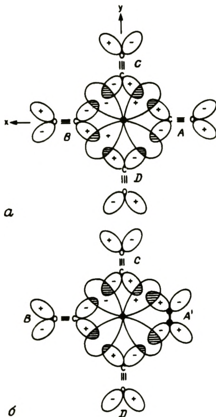
Рис. 2-7. Пример приведенной по симметрии линейной комбинации (ПСЛК) орбиталей: а) d_{xy} , ПСЛК одинаковых лигандов, \psi = \varphi_A + \varphi_B - \varphi_C - \varphi_D ; б) d_{xy} , ПСЛК трех CO и одного C_2H_4 -лигандов, \psi = \alpha\varphi_{A'} + \beta\varphi_{B'} - \gamma(\varphi_C + \varphi_D) .
