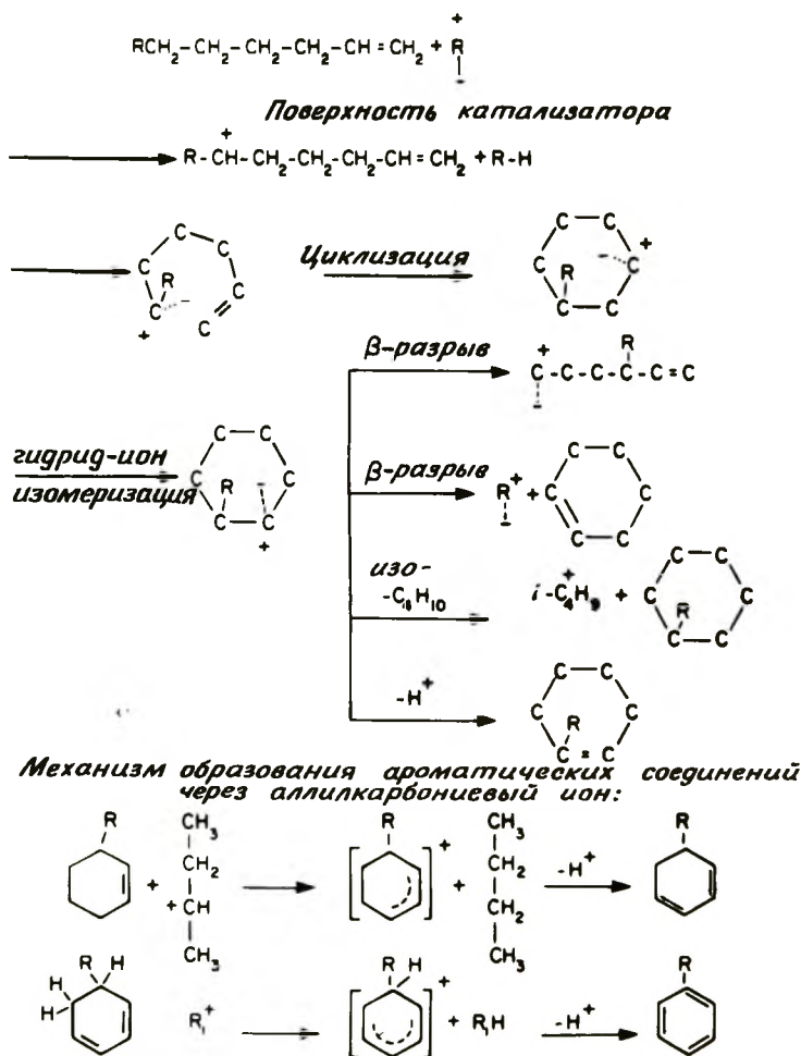
Рис. 1-14. Крекинг и изомеризация олефинов; возможные направления.
