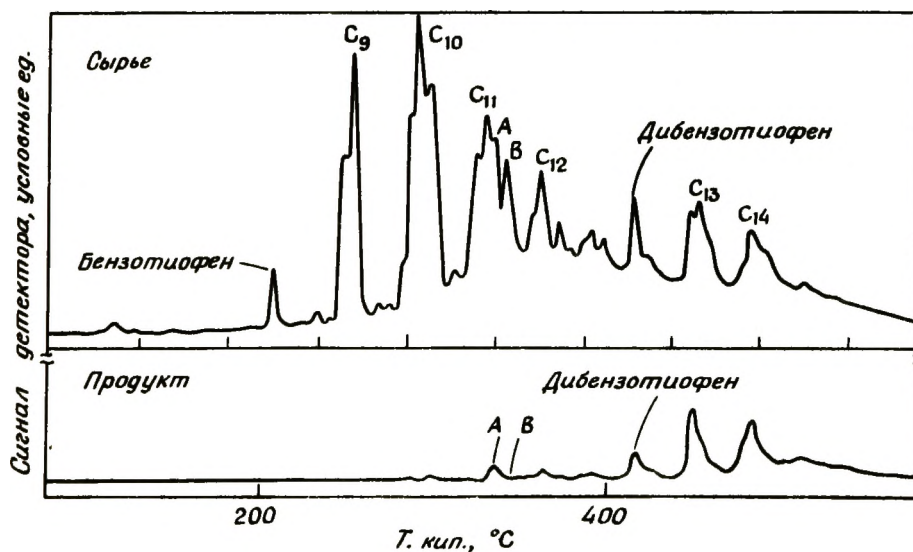
Рис. 5-4. Газохроматографические анализы бензотиофена и дибензотиофена в обессеренном и необессеренном газойле. Реакция проведена при 330°С и 20 атм [10]. (А и В — см. текст.)
