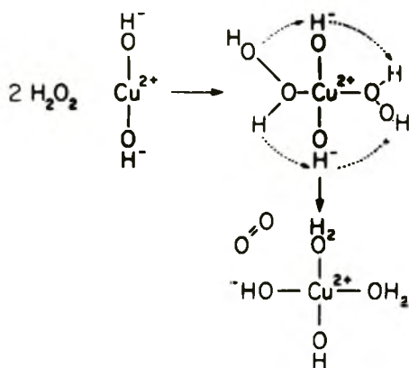
Рис. 4-6. Возможный механизм разложения \text{H}_2\text{O}_2 в присутствии \text{Cu}^{2+} .
