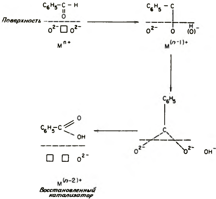
Рис. 4-9. Окисление бензальдегида на \text{SnO}_2 - \text{V}_2\text{O}_5 [14 – 15]. \square – поверхностная анионная вакансия, \text{M}^{(n-2)+} – восстановленный катализатор.
