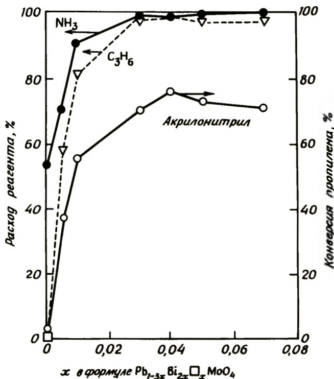
Рис. 4-14. Окислительный аммонолиз \text{NH}_3 + \text{C}_3\text{H}_6 на \text{PbMoO}_4 , промотированном \text{Bi}^{3+} [57]. [Copyright by Academic Press.]
