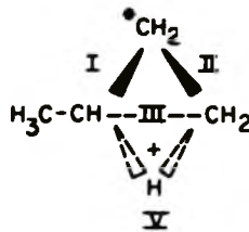
Протонированное циклопропановое кольцо при ^{13}\text{C} -изомеризации
