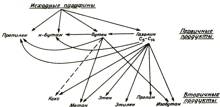
Рис. 1-25. Схема реакций, протекающих при крекинге парафинов.
