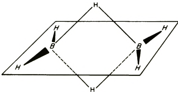
Рис. 1-7. Структура B_2H_6 . Атомы водорода, заключенные между атомами В, находятся выше и ниже плоскости, в которой лежат другие атомы.
