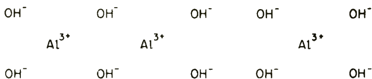
Рис. 3-43. Слои \text{Al}(\text{OH})_3 .
