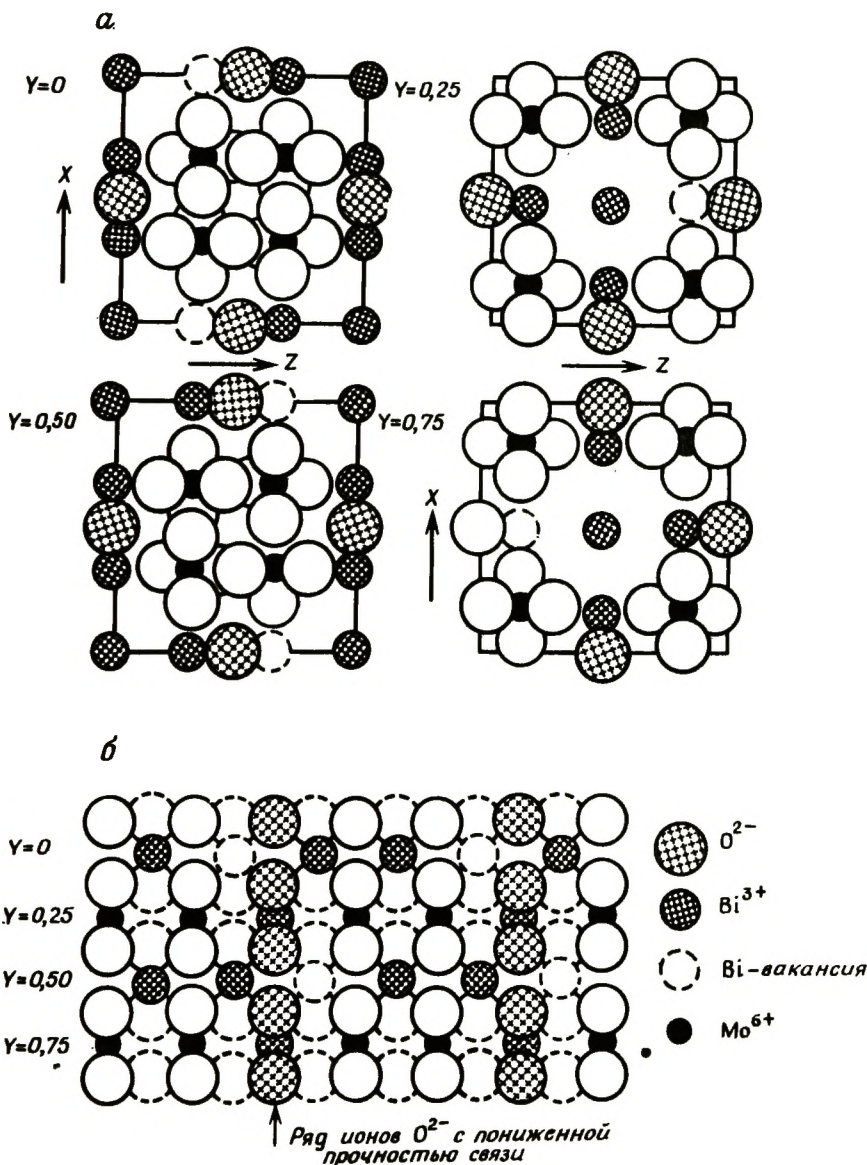
Рис. 4-28. Структура Bi_2Mo_2O_9 [83].
