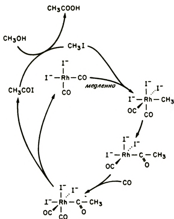
Рис. 2-21. Механизм карбонилирования метанола [36 в].
