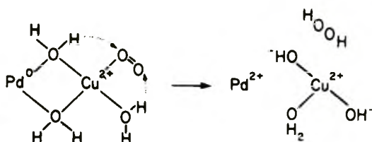
Рис. 4-7. Реокисление Pd 0 в присутствии Cu 2+ и O 2 .
