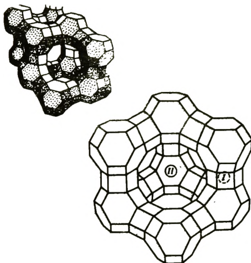
Рис. 1-34. Структура фожазита. Ионы кремния и алюминия расположены в вершинах, а ионы кислорода — вблизи ребер. I и II — типы центров; в середине — большая полость.
