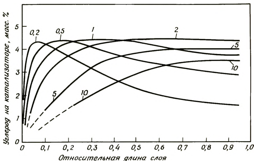
Рис. 1-23. Концентрационные профили углерода при крекинге n -гексадекана в реакторе с неподвижным слоем при различных объемных скоростях. Катализатор 13% \text{Al}_2\text{O}_3 — 87% \text{SiO}_2 ; 500^\circ\text{C} , время цикла 60 мин; числа на кривых показывают объемную часовую скорость жидкости (LHSV) [36].
