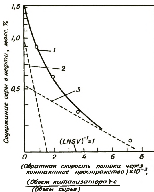
Рис. 5-8. Гидрообессеривание венесуэльского вакуумного газойля (двухкомпонентный; кинетика реакции псевдопервого порядка) [16]. 1 — общее содержание серы; 2 — превращенная фракция; 3 — непревращенная фракция.
