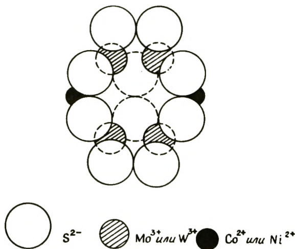
Рис. 5-14. Упрощенная модель каталитического центра для гидрообессеривания на псевдовключенной грани MoS_2 (или WS_2 ).
