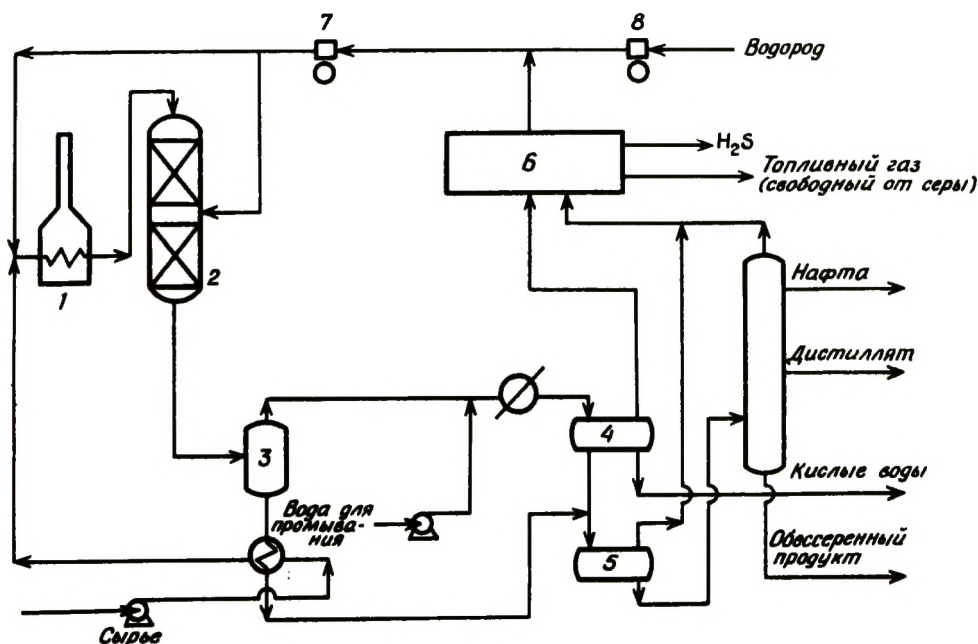
Рис. 5-17. Принципиальная технологическая схема процесса гидрообессеривания нефтяных остатков [49]. Перед главным реактором может быть установлен форконтактный реактор. 1 — котел; 2 — реактор(ы); 3, 4 — сепаратор высокого давления; 5 — сепаратор низкого давления; 6 — скруббер ( H_2S ); 7, 8 — компрессор.
