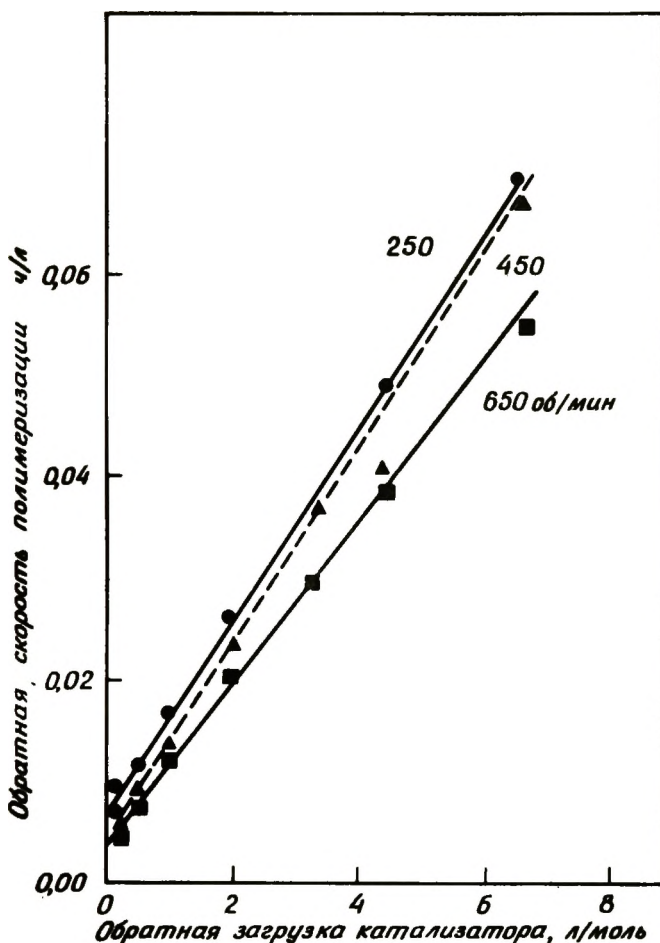
Рис. 2-42. Влияние массопереноса на скорость полимеризации этилена в реакторе с перемешиванием [40]. Условия: \text{AlEt}_2\text{Cl}=50 ммоль/л, количество \gamma\text{-TiCl}_3 увеличивали скачкообразно и соответственно каждый раз измеряли скорость; 250, 450, 650 об/мин – скорость перемешивания. [Copyright by Academic Press.]
