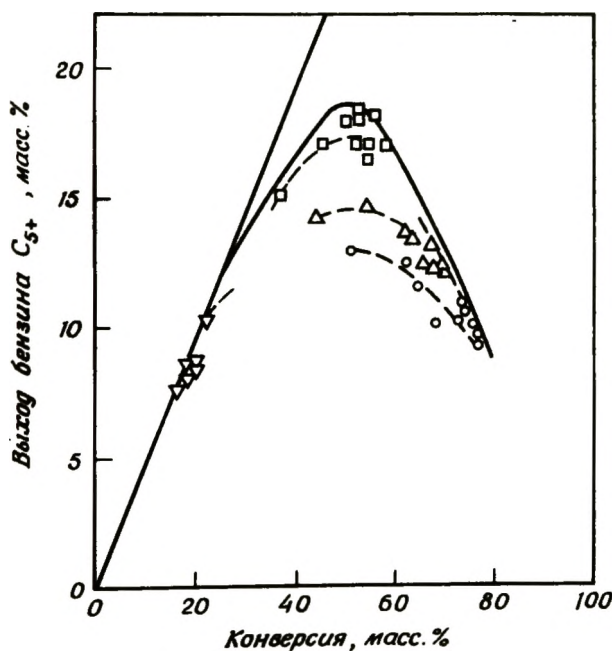
Рис. 1-16. Изменение селективности образования олефинов в бензине \text{C}_{5+} при дезактивации катализатора в реакторе с неподвижным слоем. Условия: температура 503^{\circ}\text{C} , сырье – высокопарафинистый газойль; отношение катализатор/сырье: \circ 0,25, \Delta 0,05, \square 0,01, \nabla 0,0034 [35]. [Copyright by Academic Press.] На ординате – выход олефиновой фракции \text{C}_{5+} -бензина.
