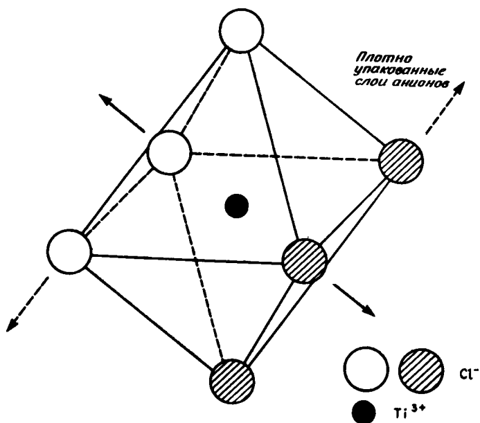
Рис. 2-33. Октаэдрические положения в слоях; сплошными стрелками показаны направления осей симметрии c_3 , перпендикулярных слоям. По отношению к этому направлению оси c_4 ориентированы под определенным углом.
