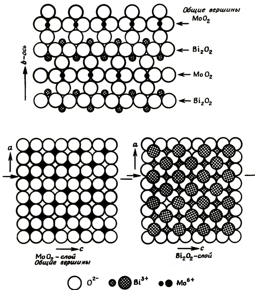
Рис. 4-26. Структура \gamma' -Bi 2 MoO 6 (коэлинит) [79, 80].
