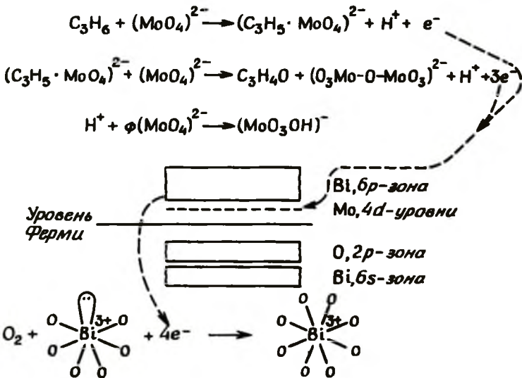
Рис. 4-17. Редокс-механизм селективного окисления пропилена на дефектах шеелитов [56а].
