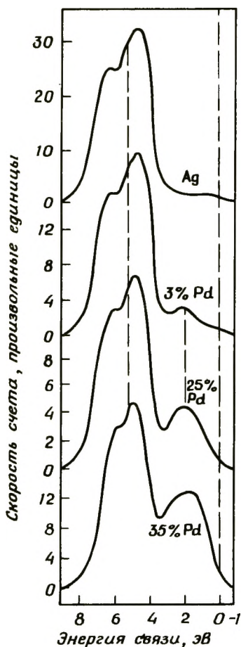
Рис. 3-24. Фотоэмиссионные спектры плотности состояний сплавов Pd – Ag [46].
