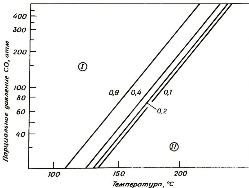
Рис. 2-17. Стабильность кобальтового катализатора [Co_2(CO)_8 + HCo(CO)_4] как функции температуры и равновесного парциального давления монооксида углерода [25]. I — стабильная область; II — нестабильная область (осаждение кобальта). 0,1, 0,2, 0,4, 0,9 — концентрация кобальта (масс, %).
