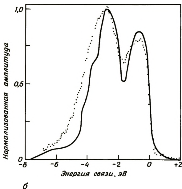
Рис. 3-23 (продолжение). а — сравнение предсказаний строгой зонной теории и теории когерентного потенциала с измеренной плотностью состояний \text{Cu}(0,6)\text{-Ni}(0,4) АВ-сплава [34]; б — данные [46] для сплава \text{Cu-Ni} .
