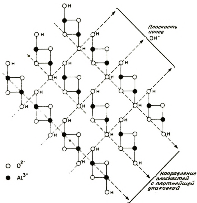
Рис. 3-45. Кристаллическая структура бемита: упаковка двойных цепей в \text{Al}(\text{OH})_3 .
