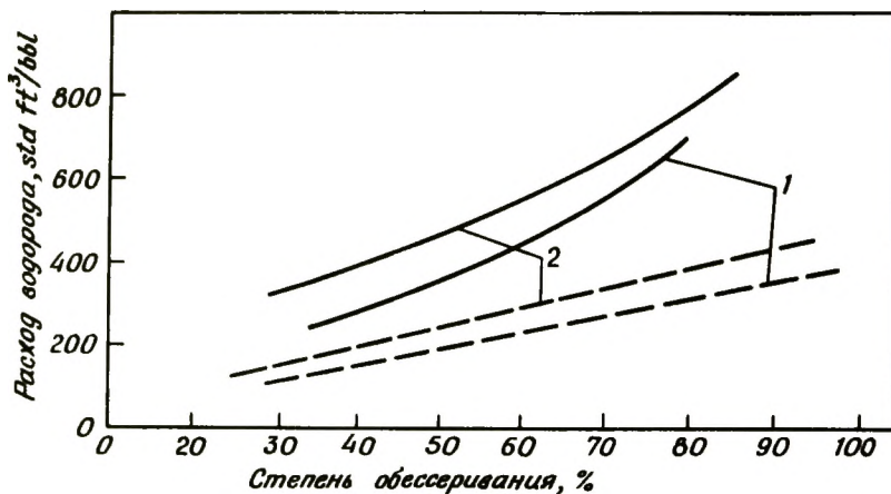
Рис. 5-19. Зависимость расхода водорода от степени обессеривания нефтяных остатков (Кувейт) [17]. — наблюдаемый расход; - - - расход, требуемый для полного удаления серы. 1 — нефтяной остаток при атмосферном давлении; 2 — вакуумный нефтяной остаток. [std — нормальные условия, НТД; 1ft (фут) = 0,3048 м; 1bbl (баррель нефтяной, США) = 158,988 дм 3 . — Перев.]
