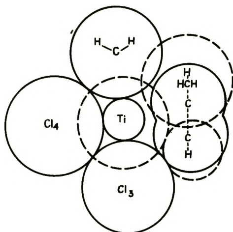
Рис. 2-35. Структура комплекса C_3H_6 с активным центром [9]. Радиусы приведены в масштабе: r_{CH_2} = 2,0 \text{ \AA} ; r_{Cl^-} = 1,8 \text{ \AA} ; r_{Ti^{3+}} = 0,8 \text{ \AA} ; r_C (в C_2H_4 ) = 1,7 \text{ \AA} .
