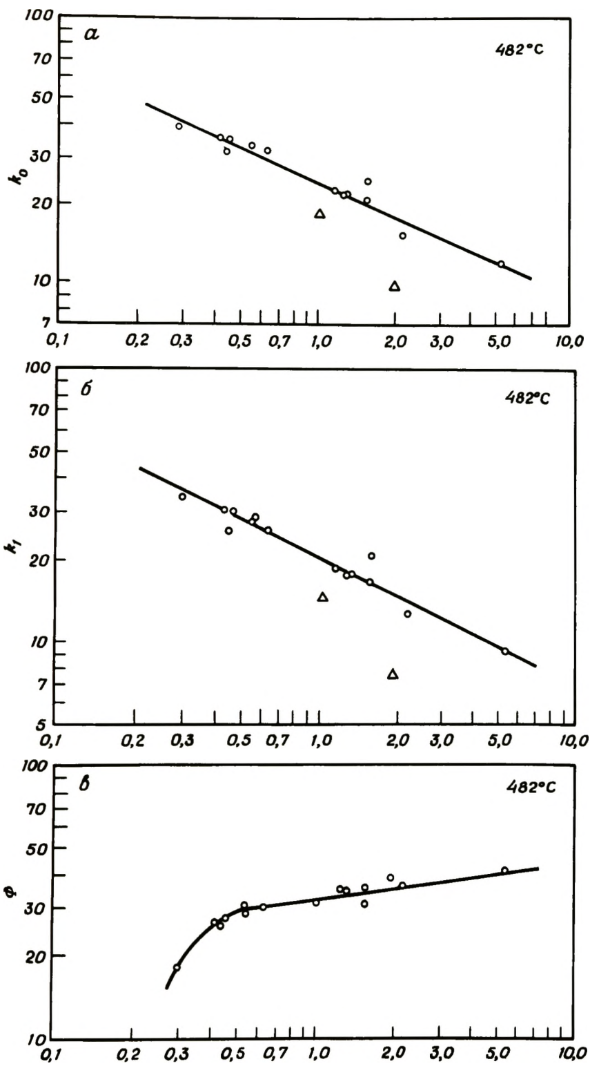
Рис. 1-61. Параметры скорости крекинга на цеолите дурабед 5 [5]. а) — константа скорости крекинга газойля; б) k_1 константа скорости образования бензина; в) \Phi — константа снижения скорости. [Copyright by the American Chemical Society.]
