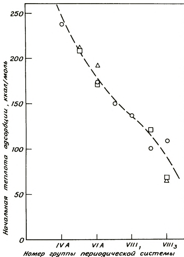
Рис. 3-10. Периодическое изменение начальной теплоты адсорбции кислорода на напыленных металлических пленках [11]. ○ элементы первого переходного периода; □ элементы второго переходного периода; Δ элементы третьего переходного периода.
