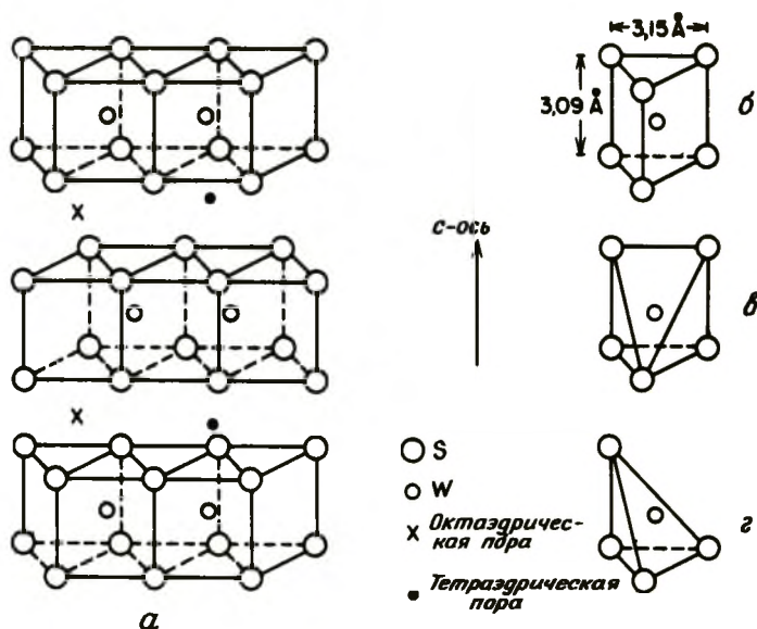
Рис. 5-10. Структура WS_2 [32]. а – упаковка слоев, иллюстрирующая положение октаэдрических пор, которые могут быть частично заняты Ni; б – симметрия окружения W^{3+} -ионов в объеме; в – на боковой грани; г – на ребре, параллельном с – оси. [Copyright by Academic Press.]
