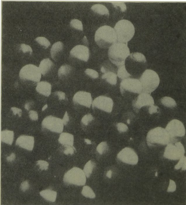
Рис. 2-39. Грань (3\bar{1}1)_2 \beta\text{-TiCl}_3 [9]. Ионы \text{Cl}^- , связанные с одним ионом \text{Ti}^{3+} , показаны в виде черных шаров.
