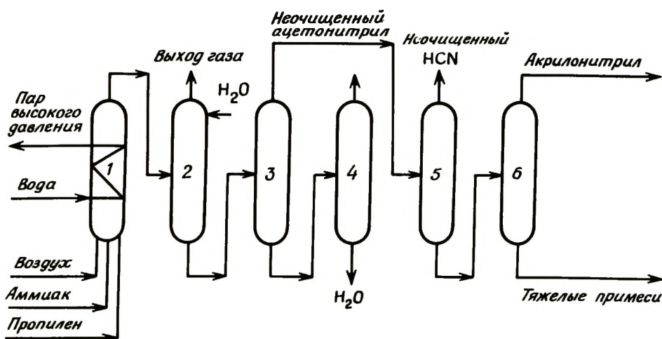
Рис. 4-31. Схема процесса окислительного аммонолиза [1]. 1 — реактор со взвешенным слоем; 2 — абсорбер; 3 — колонна извлечения акрилонитрила; 4 — колонна извлечения ацетонитрила; 5 — осветлительная колонна; 6 — колонна с продуктами.
