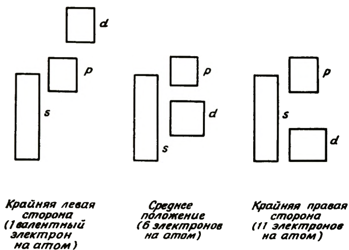
Рис. 3-6. Относительное положение s -, p - и d -зон в периоде периодической таблицы.
