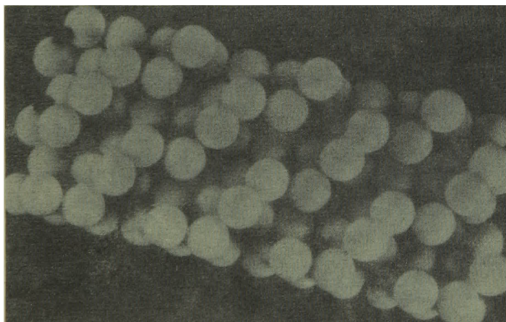
Рис. 2-34. Одна из четырех возможных структур грани (10\bar{1}0) \alpha - \text{TiCl}_3 [9]. Ионы \text{Ti}^{3+} показаны темными шариками, ионы \text{Cl}^- — белыми.
