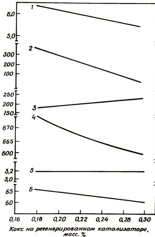
Рис. 1-63. Лифт-реактор с раздельным контролем [132]. Температура реактора 510^{\circ}\text{C} , расход сырья 66 тыс. баррелей в сутки [1 баррель нефтяной (США) = 159,988 \text{ дм}^3 ], 1 — (скорость потока воздуха) 10^{-5} л/ч; 2 — температура воздуха на входе, ^{\circ}\text{C} ; 3 — температура сырья, ^{\circ}\text{C} ; 4 — температура регенератора, ^{\circ}\text{C} ; 5 — (скорость циркуляции катализатора) \times 10^{-6} , кг/ч; 6 — конверсия, масс. %.
