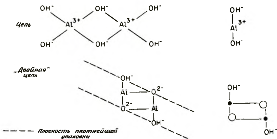
Рис. 3-44. Кристаллическая структура бемита: связь между двойным цепочечным структурным элементом в \text{AlO}(\text{OH}) и единичной цепью в \text{Al}(\text{OH})_3 .
