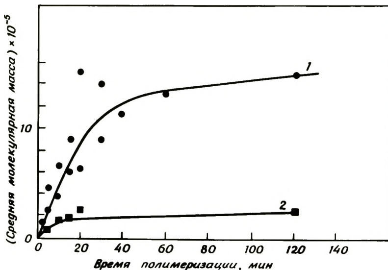
Рис. 2-31. Влияние продолжительности проведения реакции и парциального давления водорода на среднюю молекулярную массу полиэтилена [40]. Условия: 40°C, 760 мм рт. ст., [\gamma\text{-TiCl}_3] = [\text{AlEt}_2\text{Cl}] = 5,25 ммоль/л. 1 – 100% этилена; 2 – 50% этилена, 50% водорода. [Copyright by Academic Press.]
