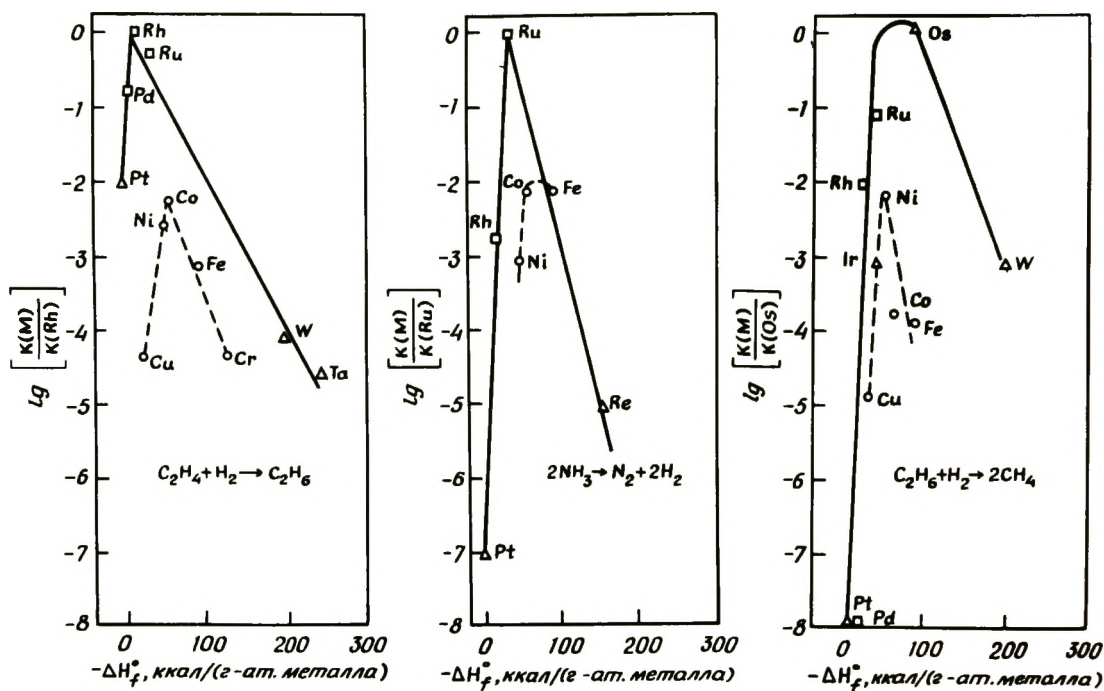
Рис. 3-16. Корреляция каталитической активности металлов согласно Танака – Тамару.
