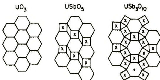
Рис. 4-19. Структуры UO_3 , USbO_5 и USb_3O_{10} .
