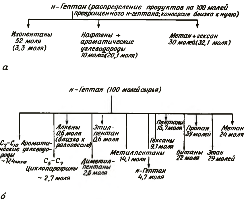
Рис. 3-57. Распределение продуктов изомеризации и гидрокрекинга n -гептана на Pt/Al_2O_3 [194]. а — на 100 молей превращаемого n -гептана в пределе, когда конверсия близка к нулю (числа в круглых скобках соответствуют количеству этих продуктов при конверсии 95,3%); б — на 100 молей сырья при 95,3% конверсии n -гептана, WHSV = 5,1 ( WHSV — см. рис. 3-52). Условия реакции: 0,6 масс.% Pt на промотированном оксиде алюминия, общее давление 34 атм, 496^\circ C , мольное соотношение H_2 : углеводород = 4,7. [Copyright by the American Chemical Society.]
