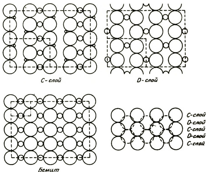
Рис. 3-48. Структура \gamma\text{-Al}_2\text{O}_3 . Показаны тетраэдрические и октаэдрические позиции иона \text{Al}^{3+} [145].
