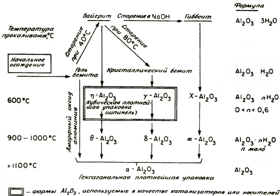
Рис. 3-39. Образование различных гидратированных форм Al_2O_3 [144, 145].
