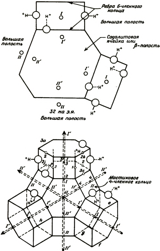
Рис. 1-37. Предполагаемое положение ионов H^+ (ОН-групп) в фожазитах. Указаны 4 различных типа кислорода. Для ясности обозначены лишь некоторые ионы H^+ . [Copyright by the American Chemical Society.]
