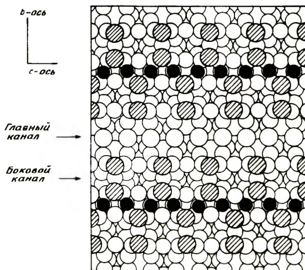
Рис. 1-38. Поперечное сечение широкого канала морденита. Видны каналы-ниши по обе стороны широкого канала; ○ атомы O, ⊗ атомы O в плоскости рисунка, ● ионы Na (некоторые из них не указаны). Al и Si в центрах каждого тетраэдра из атомов O не обозначены [60].
