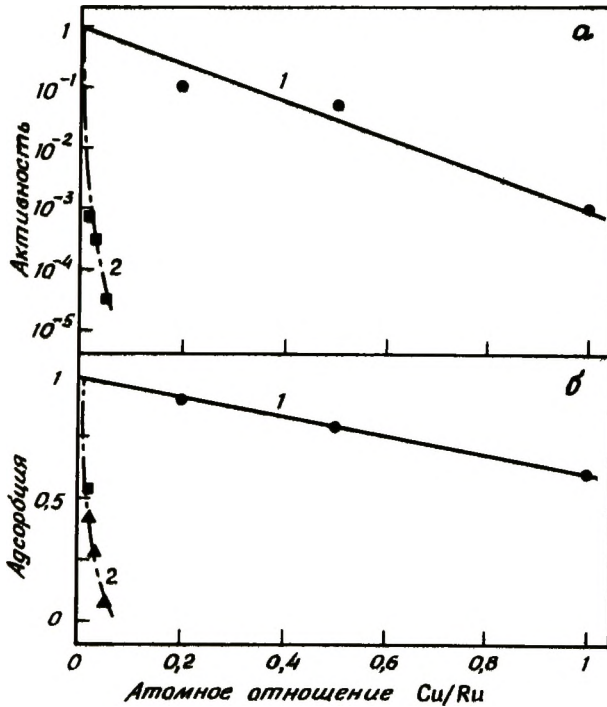
Рис. 3-76. Относительная удельная активность (а) и относительная удельная адсорбция (б) по данным Зинфельта и соотр. [Sinfelt et al., J. Catal., 42, 227 (1976)]. 1 – высокодисперсные кластеры Ru – Cu; 2 – большие частицы Ru – Cu. [Sinfelt, J. Catal., 42, 227 (1976)].
