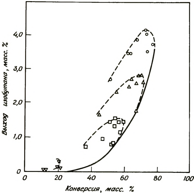
Рис. 1-19. Изменение селективности в образовании изобутана при дезактивации катализатора в реакторе с неподвижным слоем [35]. Условия те же, что на рис. 1-16. [Copyright by Academic Press.]
