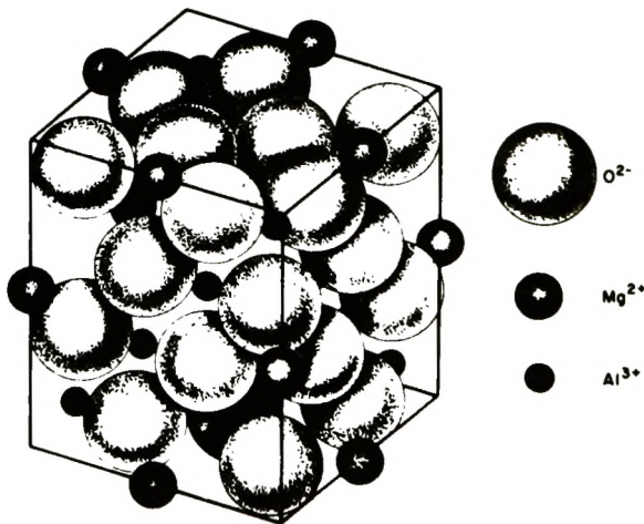
Рис. 3-46. Элементарная ячейка шпинели ( MgAl_2O_4 ) [60].
