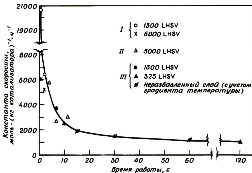
Рис. 1-54. Дезактивация катализатора \text{REnX} при образовании кокса в ходе крекинга n -гексадекана при 482^\circ\text{C} [30]. I — импульсная методика (LHSV — объемная скорость подачи сырья в 1 \text{ ч} ); II — многократные импульсы; III — непрерывный поток. [Copyright by the American Chemical Society.]
