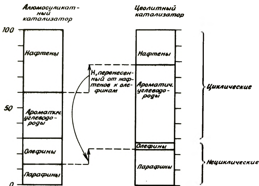
Рис. 1-52. Сравнение распределения продуктов при крекинге газойля на алюмосиликате и цеолите Y [32]. [Copyright by the American Chemical Society.]
