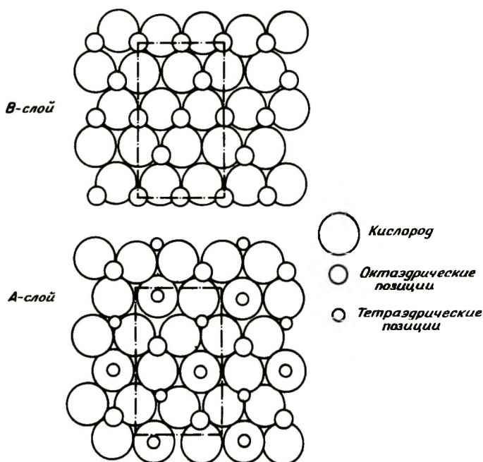
Рис. 3-47. Структура \eta\text{-Al}_2\text{O}_3 . Показаны тетраэдрические и октаэдрические положения иона \text{Al}^{3+} [145].
