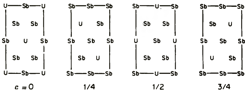
Рис. 4-20. Расположение катионов в \text{USb}_3\text{O}_{10} [13]. [Copyright by Academic Press.]
