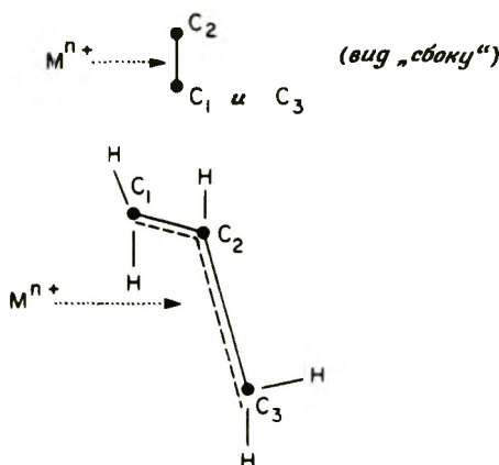
Рис. 4-10. Связывание в \pi -аллильном комплексе. I и II — схемы взаимодействия в разных проекциях, M^{n+} — ион металла.
