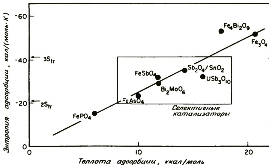
Рис. 4-13. Адсорбция бутена-1 на оксиде: зависимость энтропии адсорбции от теплоты адсорбции [53]. [Copyright by the Chemical Society (London).]
