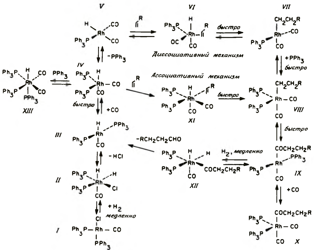
Рис. 2-18. Механизм реакции оксосинтеза, катализируемой фосфиновыми комплексами родия. Для простоты приводится только механизм, ведущий к образованию альдегида неразветвленного строения [2].
