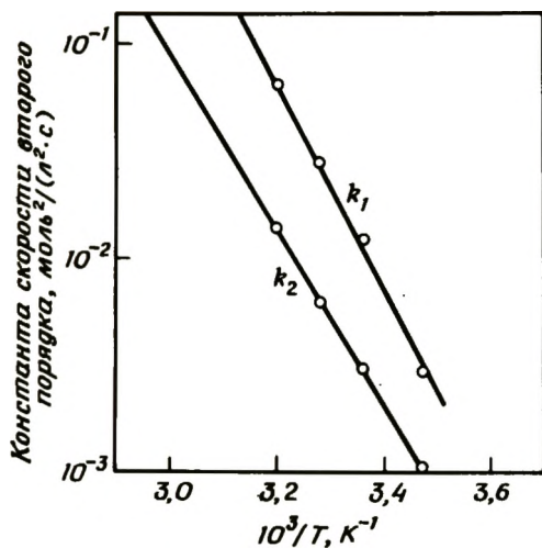
Рис. 2-11. Зависимость констант скорости окисления этилена водными растворами \text{PdCl}_4^{2-} от температуры; данные см. на рис. 2-10. Ионная сила равна 2М.
