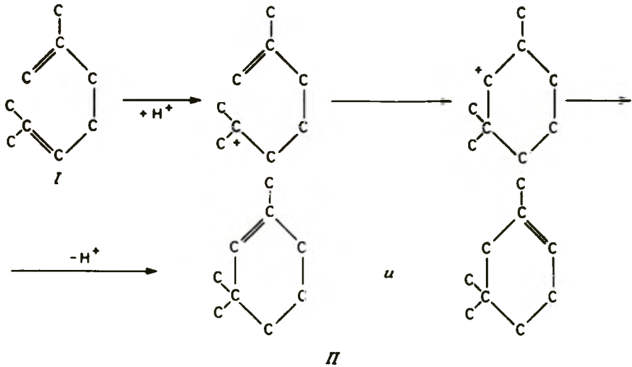
Рис. 3-56. Самоалкипирование гераниолен в серной кислоте по карбоний-ионному механизму [192]. I – гераниолен; II – циклогераниолены.
