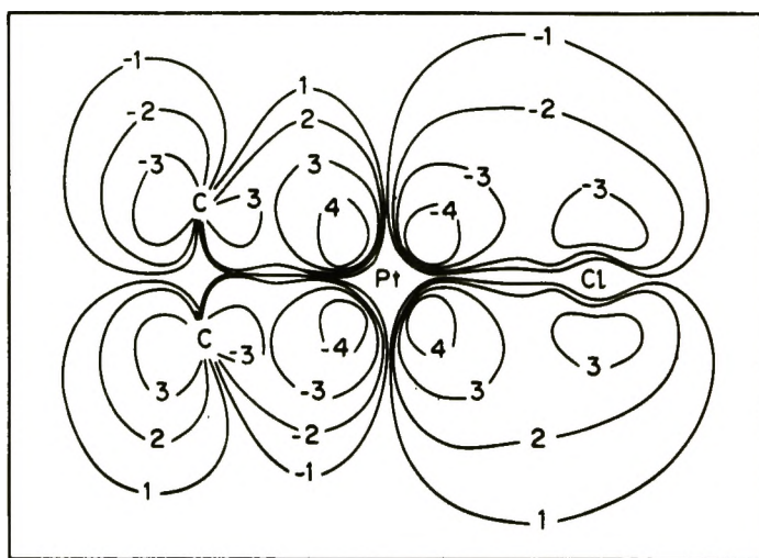
Рис. 2-9. Контуры аниона Цейзе. Волновая функция 2b_{2\pi} -связывающей орбитали иона [\text{Pt}(\text{C}_2\text{H}_4)\text{Cl}_3]^- нанесена в плоскости, образованной центральным атомом \text{Pt} , транс - \text{Cl} -лигандом и \text{C}_2\text{H}_4 -лигандом. Атомы \text{H} лежат вне этой плоскости, и их вклад в химическую связь не показан. Значения контуров даны в единицах Ридберга, а их знак определяет знак волновой функции. Внутренние узловые плоскости волновых функций вблизи каждого атома для ясности опущены [7]. [Copyright by the American Chemical Society.]
