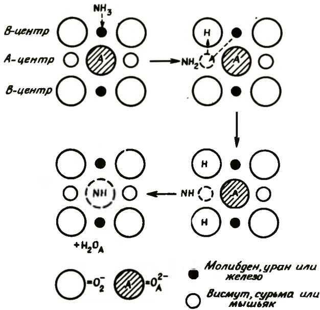
Рис. 4-16б. Механизм диссоциации аммиака на катализаторе окислительного аммонолиза согласно Матсууре. NH-группа может реагировать далее с аллилом (рис. 4-16а), давая акрилонитрил.
