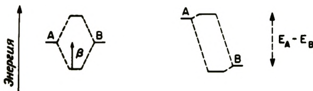
Рис. 2-5. Взаимодействие двух орбиталей \phi_A и \phi_B . Если E_A = E_B , связывающая орбиталь лежит ниже уровня E_A = E_B на расстоянии \beta , равном пространственному интегралу \int \phi_A H_0 \phi_B , где H_0 — гамильтониан. Если энергетические уровни различаются на величину E_A - E_B , связывающая орбиталь лежит ниже уровня B примерно на \beta / (E_A - E_B) .
