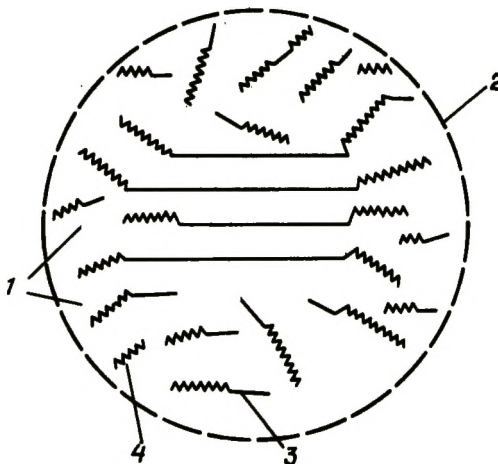
Рис. 5-24. Схематическое изображение асфальтена [60]. [Copyright by the American Chemical Society.] 1 – смолообразные молекулы; 2 – нечетко выраженный край, за пределами которого – межмицеллярная жидкость; 3 – конденсированные ароматические фрагменты; 4 – углеродные цепи или нафтеновые фрагменты.
