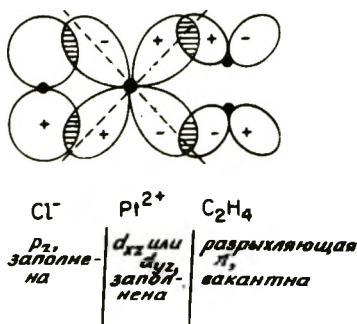
Рис. 2-8. Линейное расположение иона Pt^{2+} и лигандов Cl^- и C_2H_4 .
