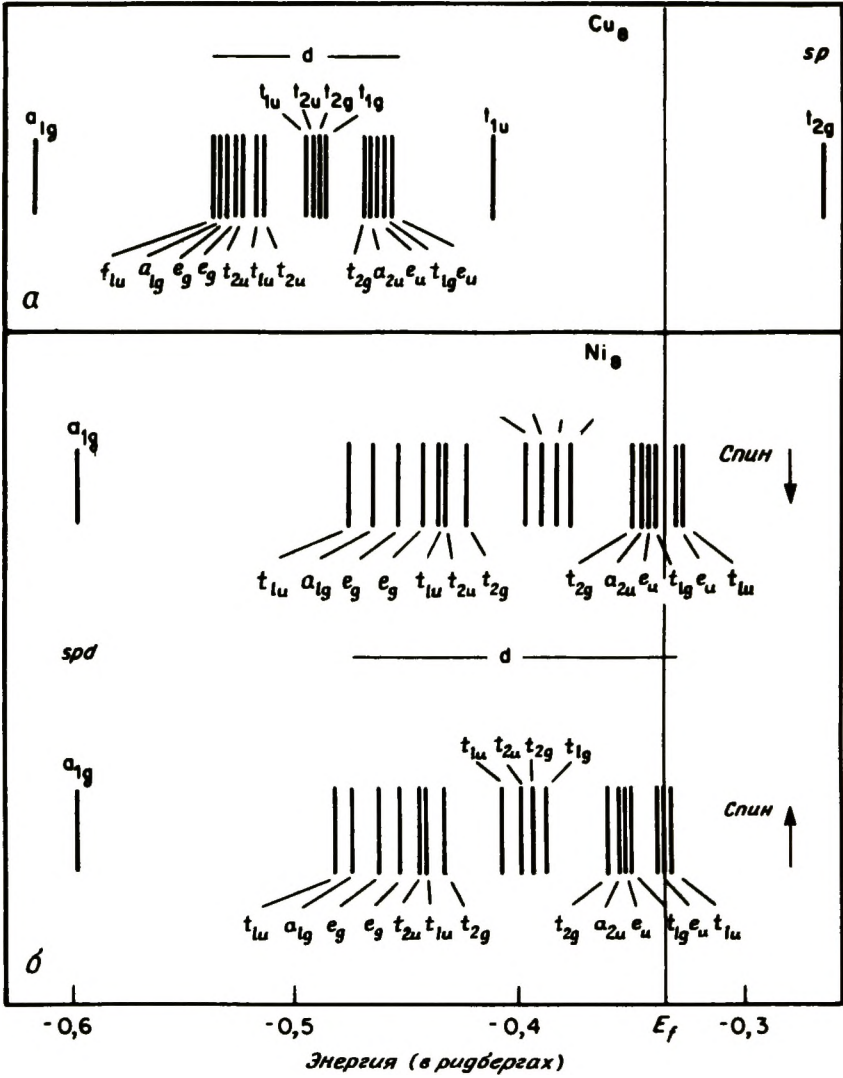
Рис. 3-31. Энергетические уровни кластеров Cu и Ni. а – электронные энергетические уровни на основе модели ССП- \chi\alpha для кубического кластера Cu 8 ; б – спин-поляризованные энергетические уровни ССП- \chi\alpha кубического кластера Ni 8 . Для каждого кластера результаты показаны с учетом того, что межъядерное расстояние между ближайшими соседними атомами равно расстоянию в объеме кристалла [62]. [Copyright by the American Institute of Physics.]
