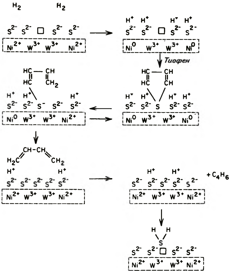
Рис. 5-15. Предполагаемый механизм гидрообессеривания тиафена. □ анионная вакансия; штриховой прямоугольник означает, что на включенных катионах могут находиться (частично) делокализованные электроны.
