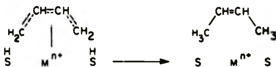
Рис. 5-16. Предполагаемые механизмы гидрогенизации олефинов на сульфидированных катализаторах. В промежуточном соединении образуется с поверхностью \sigma -связь (а) или \pi -связь (б).
