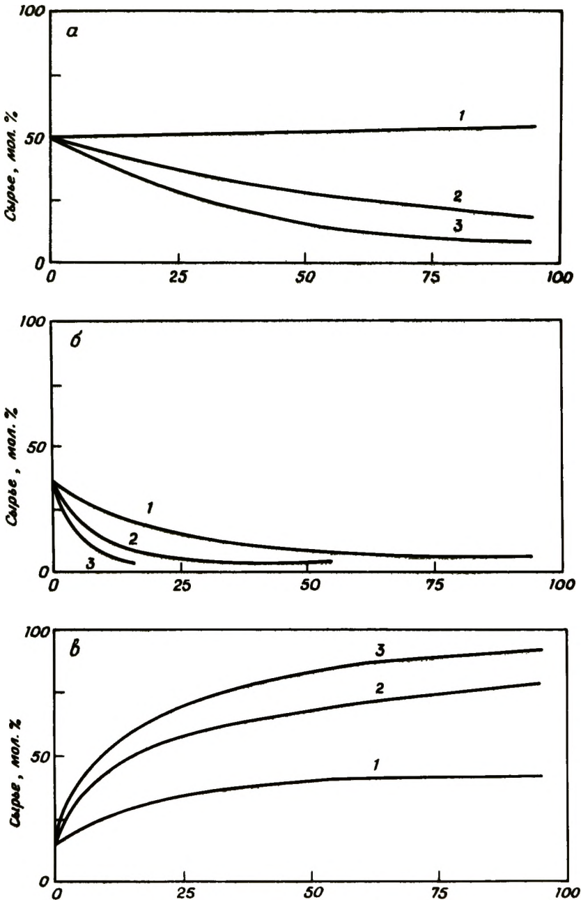
Рис. 3-71. Рассчитанная конверсия нефти с использованием минимального (1), среднего (2) и максимального (3) значений констант скорости первого порядка. Условия реакции указаны в табл. 3-18. а – средние парафины, общее значение k ; б – нафтены, общее значение k ; в – ароматические углеводороды, общее значение k .
