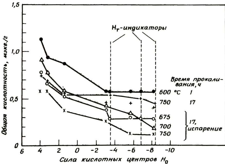
Рис. 1-50. Влияние температуры прокалывания и условий обработки паром на распределение кислотных центров по силе в цеолите REY [39]. [Copyright by Academic Press.]
