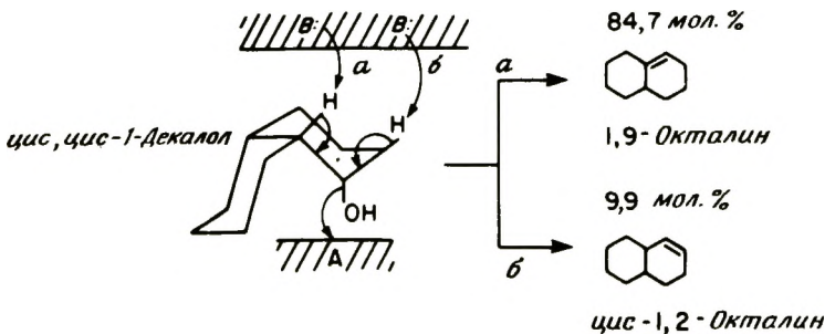
Рис. 1-10. Предполагаемый механизм дегидратации цис,цис -1-декалопа на оксиде алюминия [28]. Схема реакции объясняет преобладание направления a — транс -элиминирования. A — кислотный центр; B — основной центр. [Copyright by Academic Press.]
