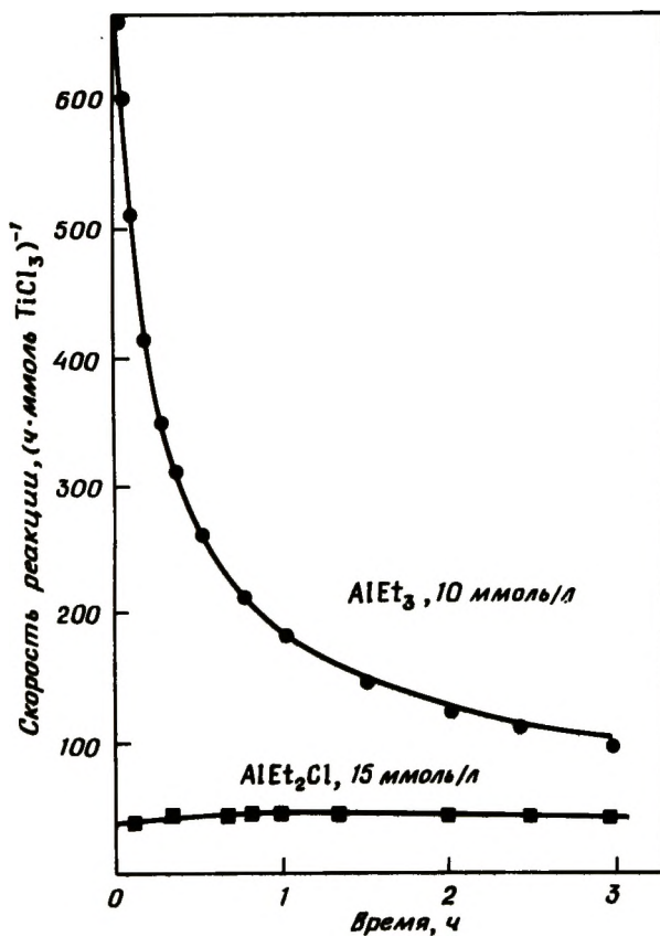
Рис. 2-25. Влияние состава алкилалюминия на стабильность катализатора. Условия: 80^{\circ}\text{C} , \text{TiCl}_3 в ундекане, без \text{H}_2 . Полагают, что мономер — это этилен [40]. [Copyright by Academic Press.]
