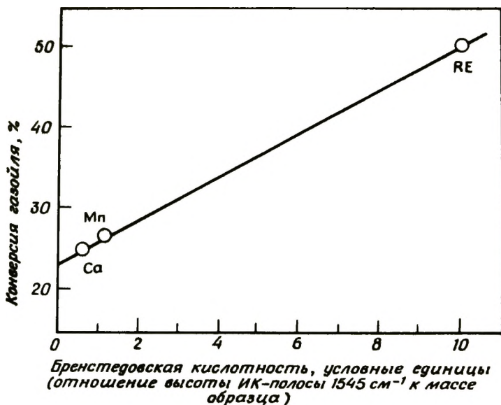
Рис. 1-44. Корреляция между каталитической активностью в крекинге газойля и брэнстедовской кислотностью Ca-, Mn- и REX-цеолитов [94]. [Copyright by Academic Press.]
