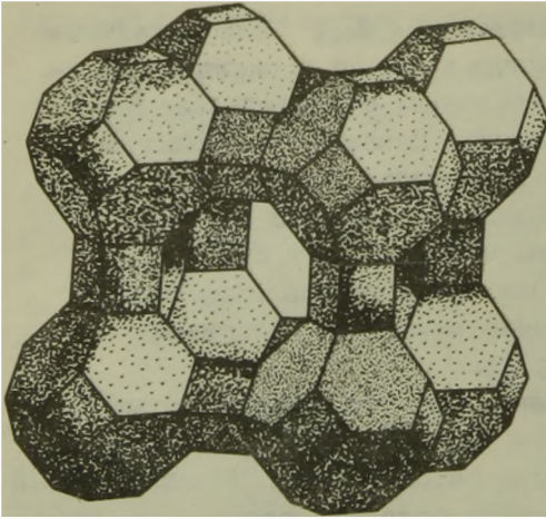
Рис. 1-32. Размещение усеченных октаэдров в цеолите А.
