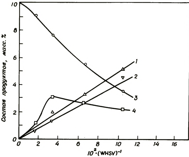
Рис. 3-52. Реакция n -гексана на Pt, нанесенной на неокислотный оксид алюминия. Условия реакции: температура 440°C; давление 9,5 атм; мольное соотношение \text{H}_2 : n\text{C}_6 = 4 ; катализатор — 0,5 масс. % Pt на неокислотном \text{Al}_2\text{O}_3 [136]. 1) 0,2 \times изо- \text{C}_6 ; 2) бензол; 3) 0,10 \times n\text{-C}_6 ; 4) метилциклопентан. WHSV — массовая скорость потока через контактное пространство в час. [Copyright by Academic Press.]
