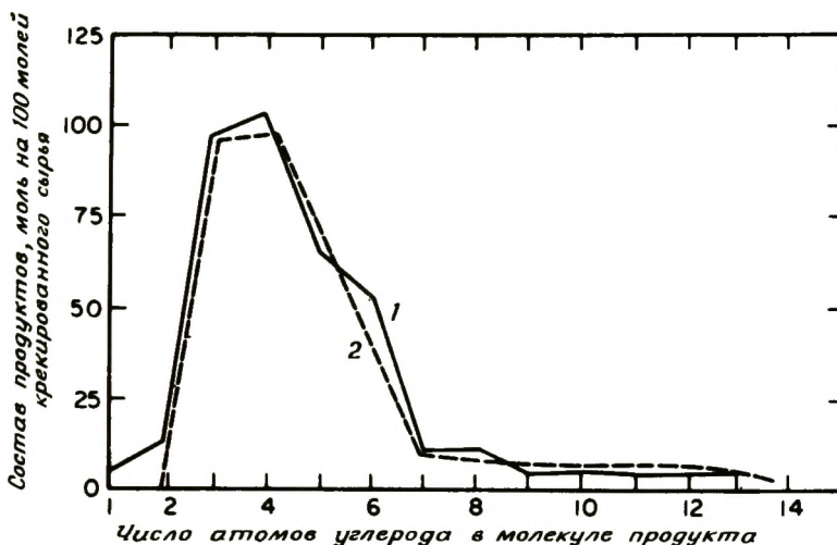
Рис. 1-13. Каталитический крекинг n -гексадекана. 1 — экспериментальные данные по составу продуктов при 24% конверсии в присутствии катализатора \text{SiO}_2 - \text{ZrO}_2 - \text{Al}_2\text{O}_3 при 500^\circ\text{C} и объемной скорости \text{LHSV} = 10 ; 2 — распределение продуктов, рассчитанное по правилам, приведенным в тексте [6, 10]. [Copyright 1958 by Litton Educational Publishing Company.]
