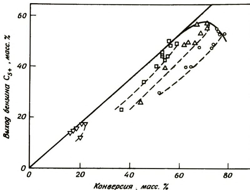
Рис. 1-15. Изменение селективности образования бензина при дезактивации катализатора в реакторе с неподвижным слоем. Условия: температура 503^{\circ}\text{C} , сырье – высокопарафинистый газойль; отношение катализатор/сырье: \circ 0,25, \Delta 0,05, \square 0,01, \nabla 0,0034 [35]. [Copyright by Academic Press.]
