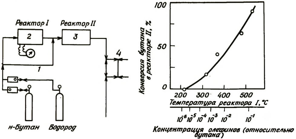
Рис. 1-12. Аппаратурная схема и график, показывающий роль олефинов в иницировании крекинга бутана [32]. [Copyright by the American Chemical Society.] 1 — байпас; 2 — Pt-катализатор; 3 — катализатор морденит; 4 — петля для отбора проб.
