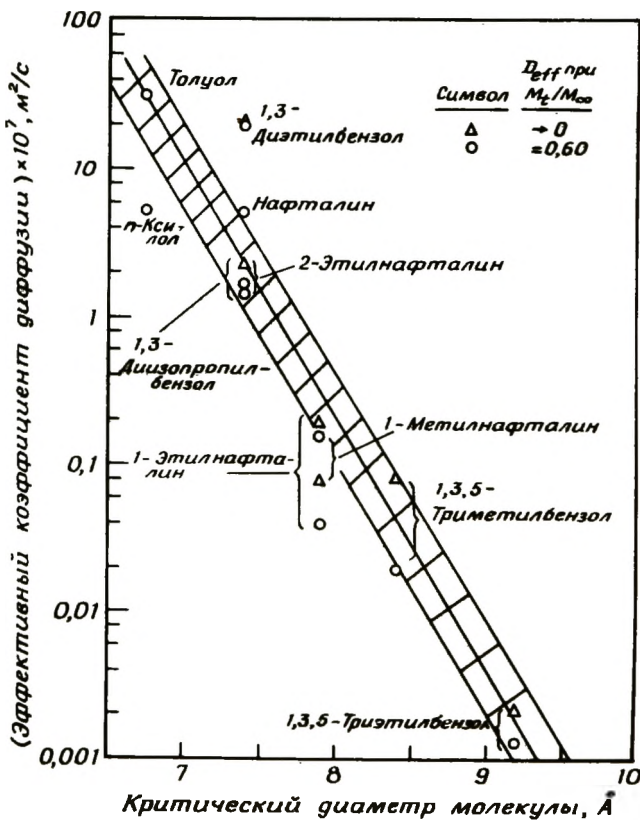
Рис. 1-55. Зависимость эффективного коэффициента диффузии от критического диаметра диффундирующей молекулы. Адсорбционная контрдиффузия в насыщенный циклогексаном NaY при 25°C; свободный диаметр пор равен 7,4 Å. M_t/M_\infty характеризует близость к равновесию [120].
