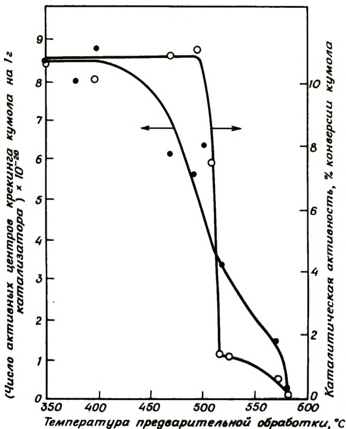
Рис. 1-47. Влияние температуры предварительной обработки цеолита NaHY на концентрацию брэнстедовских кислотных центров и активность в крекинге кумола при 325°C [98]. [Copyright by the American Chemical Society.]
