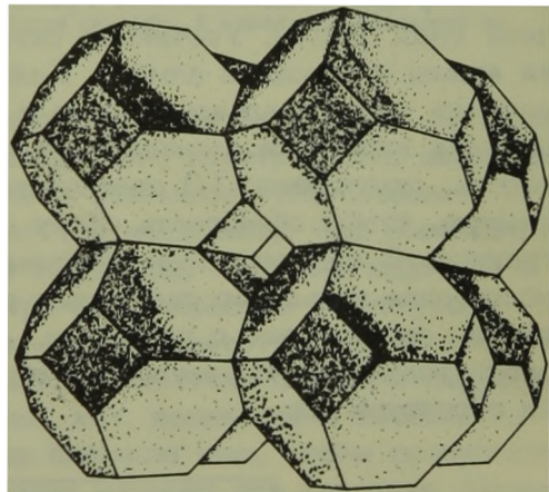
Рис. 1-31. Размещение усеченных октаэдров в содалите.
