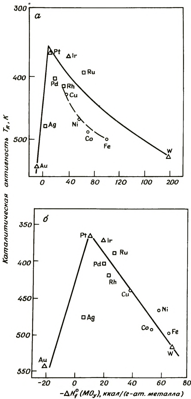
Рис. 3-15. Каталитическая активность металлов в разложении муравьиной кислоты по Танака – Тамару (а) и Захтлеру – Фаренфорту (б). Параметр Танака – Тамару определялся как теплота образования высшего устойчивого оксида на 1 моль металла. Параметр Захтлера – Фаренфорта определялся как теплота образования наиболее устойчивого оксида металла на 1 моль кислорода.
