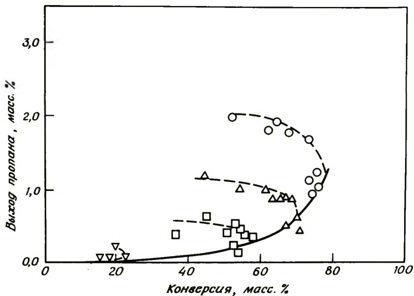
Рис. 1-20. Изменение селективности в образовании пропана при дезактивации катализатора в реакторе с неподвижным слоем [35]. Условия те же, что на рис. 1-16. [Copyright by Academic Press.]
