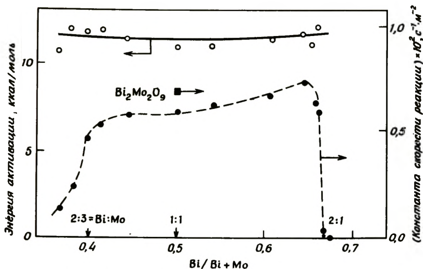
Рис. 4-29. Активность висмутмолибдатных катализаторов в окислении бутена [88].
