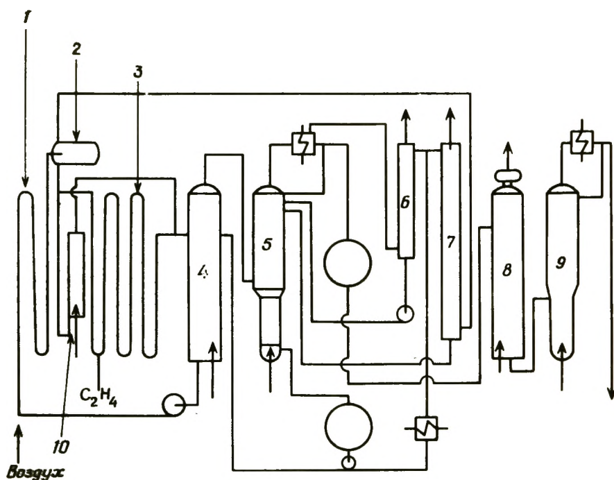
Рис. 2-13. Двухреакторная схема вакуум-процесса. Регенератор используется для разложения побочного продукта — оксалата меди [14]. 1 — трубчатый реактор для повторного окисления \text{Cu}^+ ; 2 — фазовый сепаратор; 3 — трубчатый реактор образования альдегида; 4 — испарительная колонна; 5, 9 — перегонка; 6, 7 — скрубберы; 8 — обезгаживание; 10 — регенератор. [Copyright by the American Chemical Society.]
