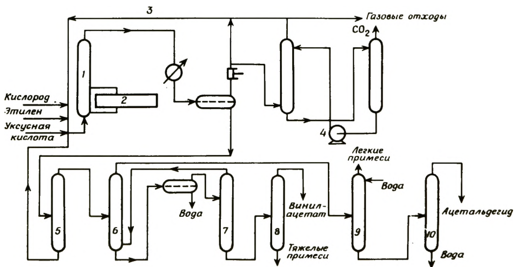
Рис. 2-16. Принципиальная технологическая схема синтеза винилацетата [19]. 1 - реактор; 2 - регенерация; 3 - рециркуляция; 4 - отделение \text{CO}_2 ; 5 - регенерация уксусной кислоты; 6 - отделение ацетальдегида; 7 - отделение воды; 8 - дистилляция винилацетата; 9 - поглощение ацетальдегида; 10 - дистилляция ацетальдегида.
