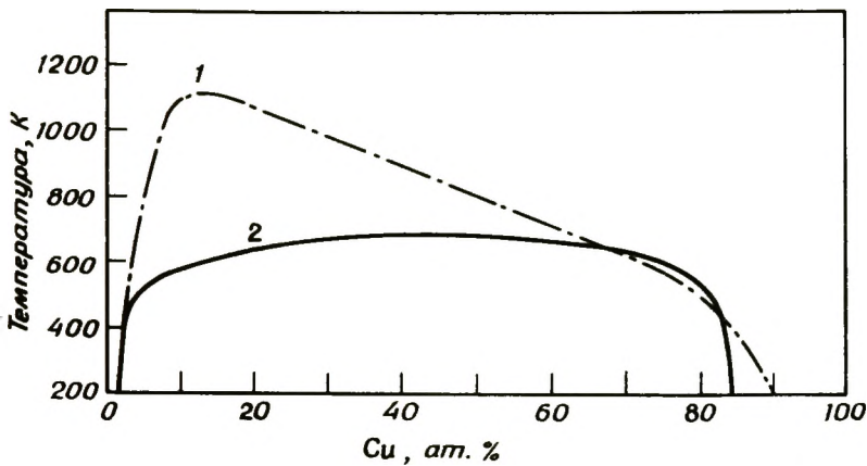
Рис. 3-20. Фазовая диаграмма для системы Cu – Ni, рассчитанная из термодинамических данных [35a] (1) и [35б] (2). [Copyright by Academic Press.]
