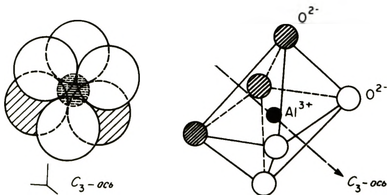
Рис. 3-41. Октаэдрическое положение иона \text{Al}^{3+} .
