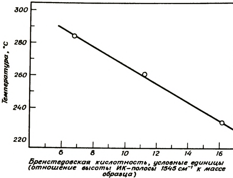
Рис. 1-46. Корреляция между каталитической активностью (измеренной как температура, необходимая для 25% конверсии o -ксилола) и брэнстедовской кислотностью цеолита Y, содержащего катионы редкоземельных элементов [96]. [Copyright by Academic Press.]
