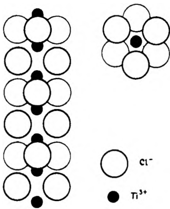
Рис. 2-38. Расположение ионов в \beta\text{-TiCl}_3 .
