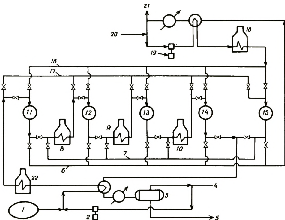
Рис. 3-4. Схема циклической установки для реформинга с регенерацией. Верхний и нижний коллекторы реакторов имеют несколько выводов, так что каждый из реакторов может быть поставлен на регенерацию, в то время как остальные объединены в единую установку, работающую в оптимальном режиме. 1 - сырье; 2 - компрессор рециркулирующего газа; 3 - сепараторный барабан; 4 - H_2 высокой очистки; 5 - реформат к стабилизатору; 6 - нижний коллектор регенерации; 7 - нижний реакционный коллектор; 8 - первый повторный подогрев; 9 - второй повторный подогрев; 10 - третий повторный подогрев; 11 - 14 - реактор; 15 - качающийся реактор; 16 - верхний коллектор регенерации; 17 - верхний реакционный коллектор; 18 - предварительный подогрев топливного газа; 19 - компрессор рециркулирующего топочного газа; 20 - воздух или топочный газ; 21 - избыточный газ; 22 - печь предварительного подогрева.
