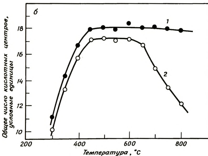
Рис. 1-43. Относительная концентрация брэнстедовских и льюисовских кислотных центров цеолита Y по данным ИК-спектроскопии [92]. а – интенсивность ИК-полос поглощения пиридина, хемосорбированного на брэнстедовских и льюисовских кислотных центрах цеолита Y, как функция температуры предварительной активации (1 – брэнстедовские центры, 2 – льюисовские центры); б – общая кислотность как функция температуры предварительной активации (1 – брэнстедовская кислотность плюс удвоенная льюисовская кислотность, 2 – брэнстедовская кислотность плюс льюисовская кислотность). [ Copyright by Academic Press.]
