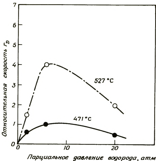
Рис. 3-63. Влияние парциального давления водорода на относительную скорость дегидроциклизации n -гептана на катализаторе Pt/Al 2 O 3 [203]. P_{H-C_7} = 1,2 атм. r_D — скорость относительно скорости дегидроциклизации при 471°C и парциальном давлении водорода 5,8 атм на том же катализаторе. [Copyright by the American Chemical Society.]
