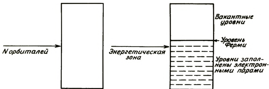
Рис. 3-5. Образование энергетической зоны при сочетании орбиталей и размещение в этой зоне электронных пар.
