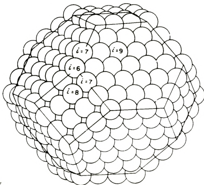
Рис. 3-38. Расположение поверхностных атомов в гранцентрированном кубическом кристаллите [121]. а – октаэдрическая конфигурация; б – кубооктаэдрическая конфигурация. Значения i определяют номер ближайших соседей.
