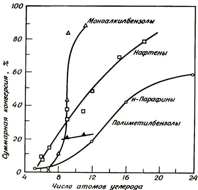
Рис. 1-11. Сравнение различных классов углеводородов в процессе каталитического крекинга. Условия реакции: катализатор Al_2O_3 - ZrO_2 - SiO_2 ; 500°С; 13,7 молей углеводородного сырья на 1 л катализатора в 1 ч; приведена суммарная активность за 1 ч работы, т.е. усредненная величина, так как катализатор в процессе работы дезактивируется [6]. [Copyright 1958 by Litton Educational Publishing Company.]
