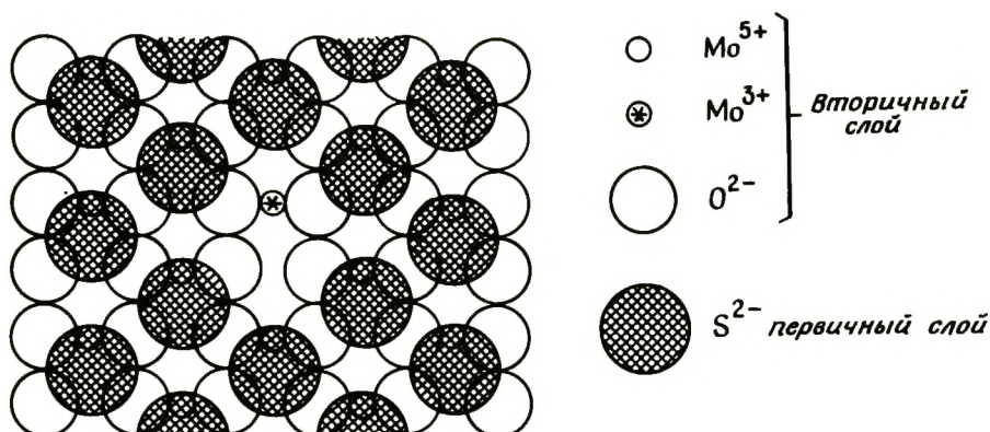
Рис. 5-9а. Сульфированные монослои на \gamma-Al_2O_3 , промотированном Со; поверхностный слой представляет собой С-слой [12].
